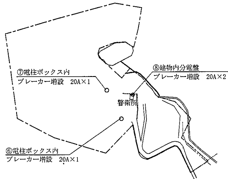
大塚山地区配置図 S=NS
