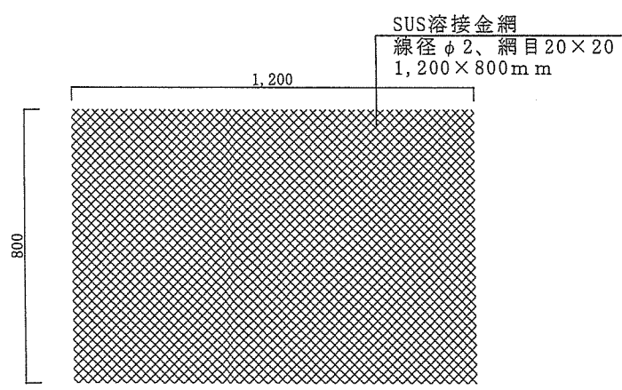
し渣ゲート金網詳細図 S=1/20
