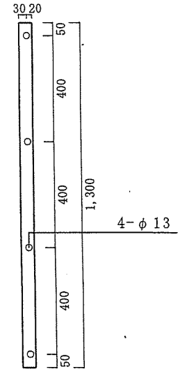
し渣ゲート枠詳細図 S=1/20
