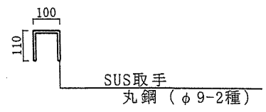
取手詳細図 S=1/20
