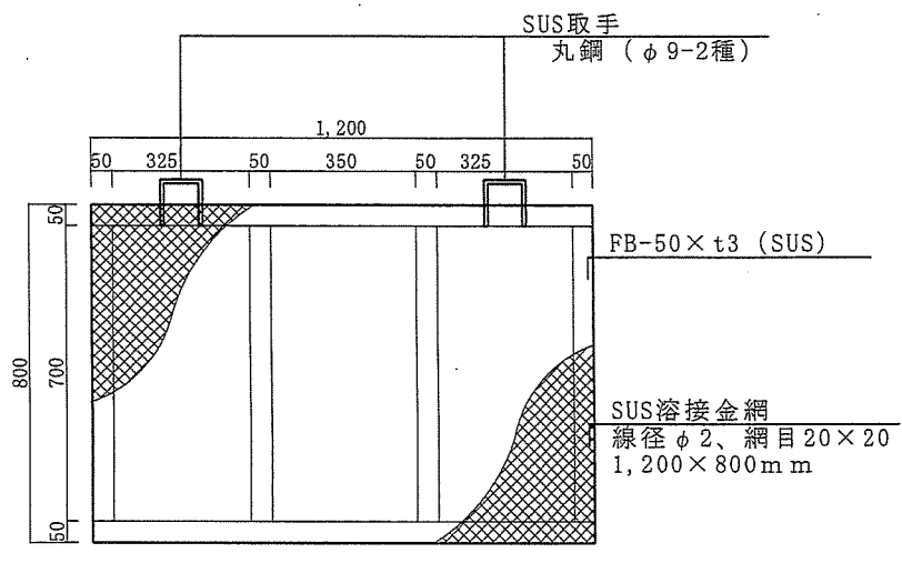
し渣ゲート詳細図 S=1/20
