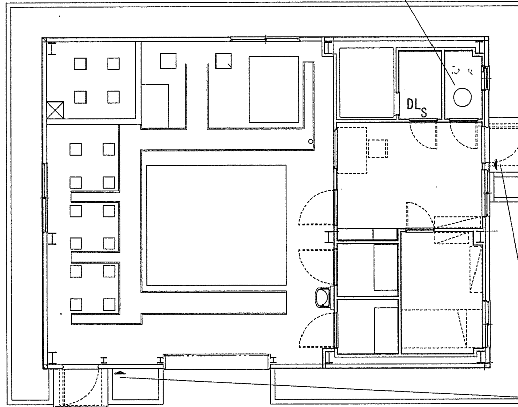
28号ボイラー室平面図
