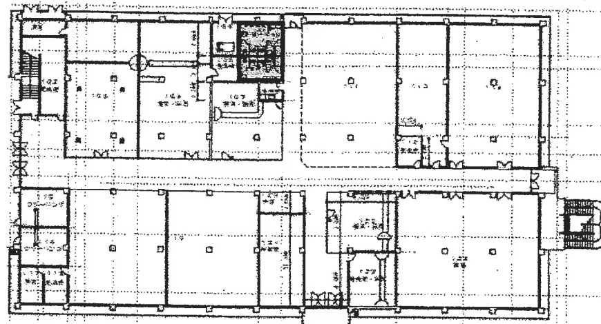
115号建物平面図
