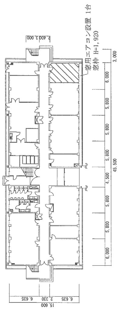
30号建物1階平面図 S=1/600
