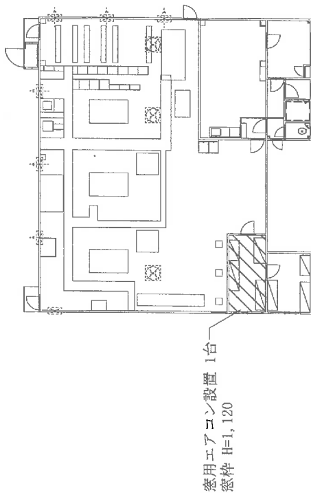
15号建物平面図 S=1/200
