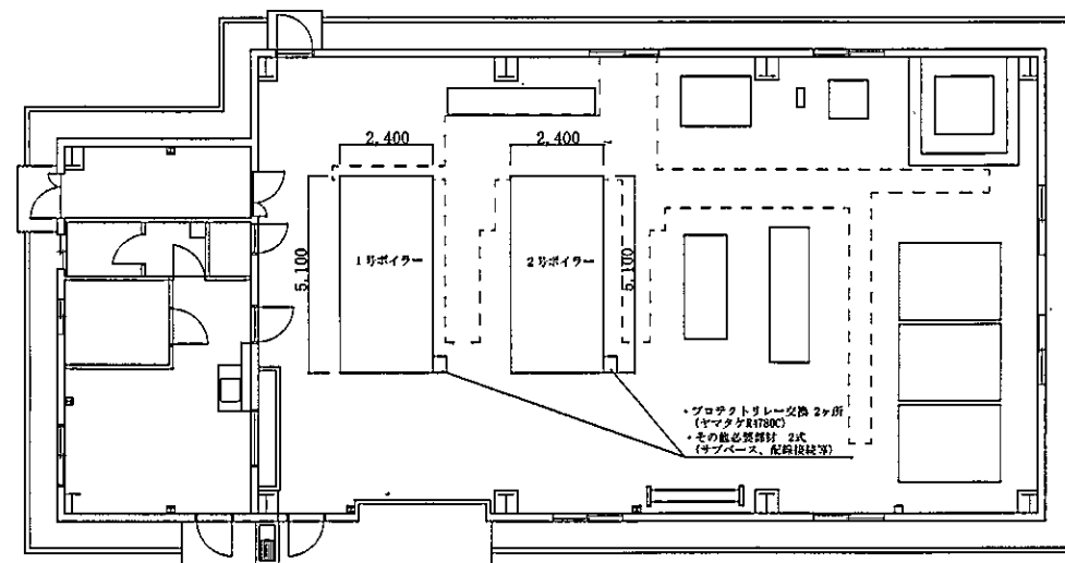
平面図 S=1/150
