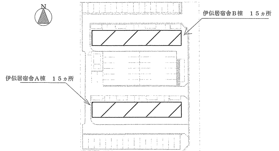
伊伝居宿舎A/B棟配置図 S=1/1,000
