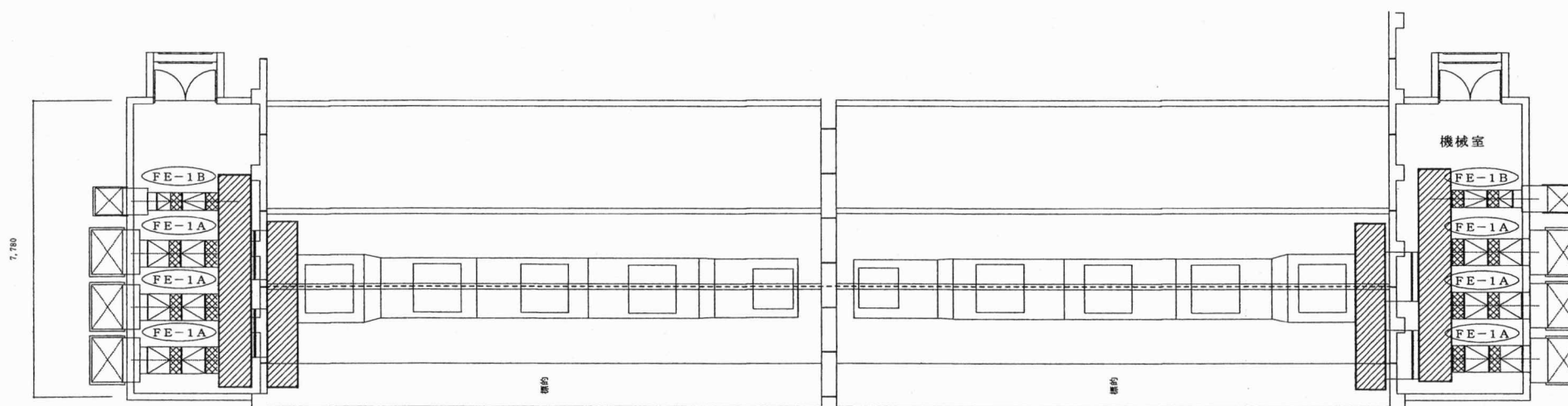
平面図 (100m射座及び25m) S=1/150
