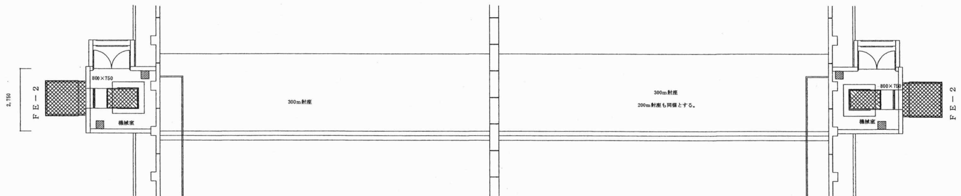
平面図 (300m射座) S=1/150
