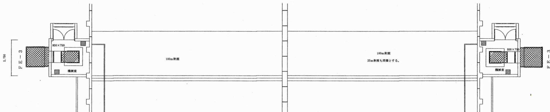
平面図 (100m射座及び25m) S=1/150
