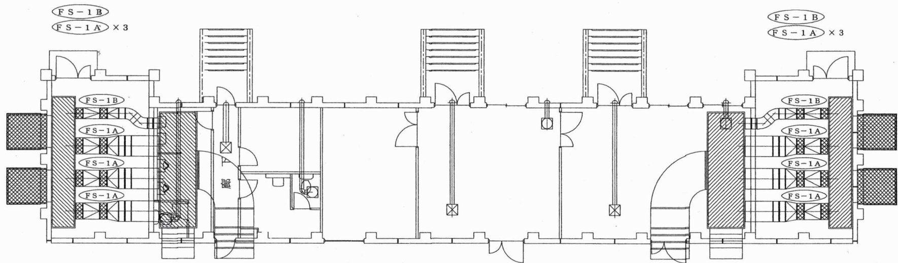
日野訓練場換気設備平面図 S=1/150
