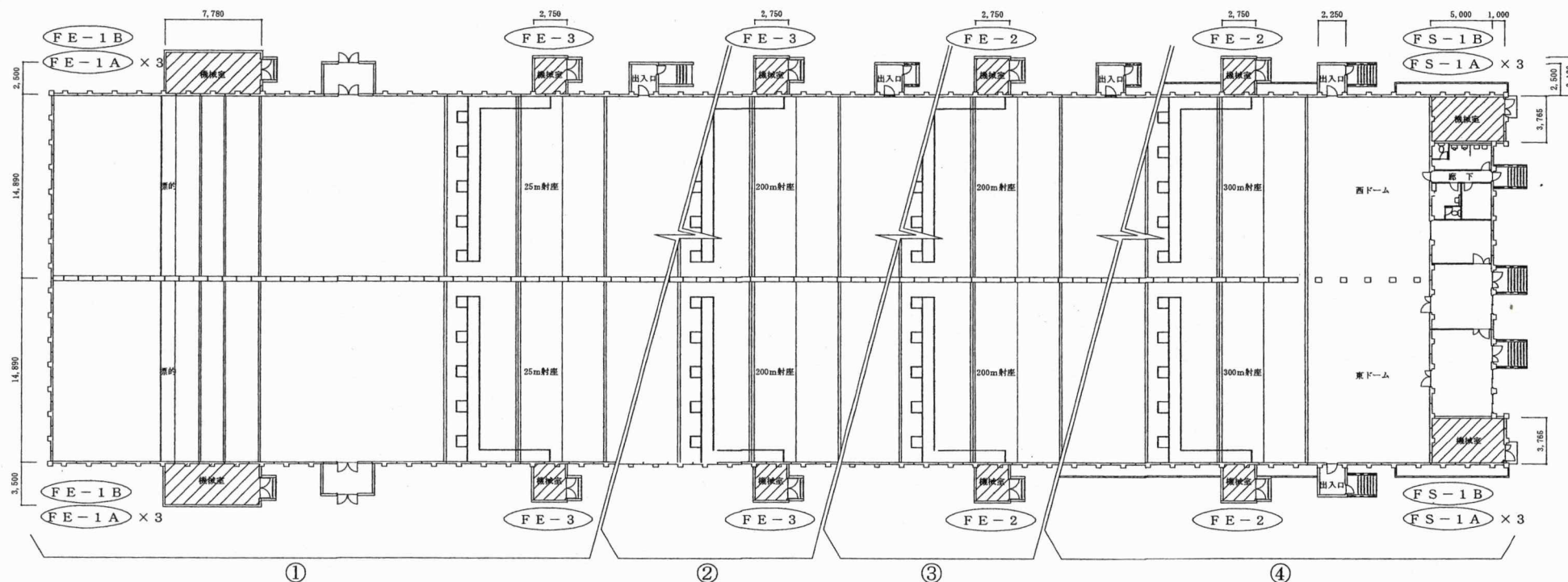
日野訓練場換気設備平面図 S=1/500
