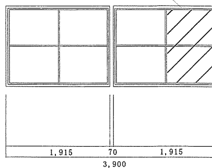
88号建物2階会議室 建具図 S=1/50
