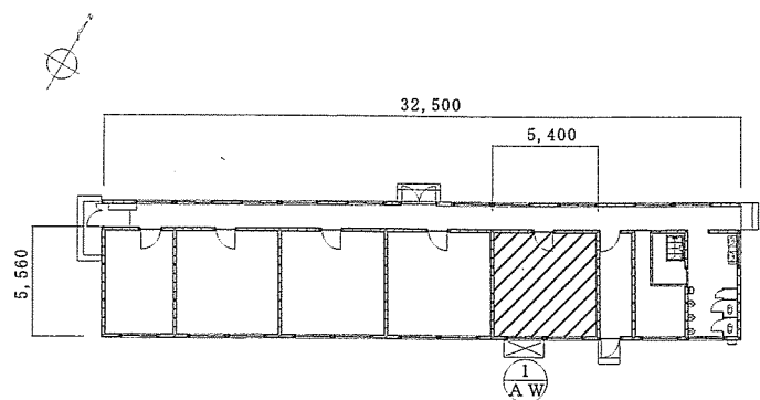
6号建物 平面図 S = 1 / 3 0 0
