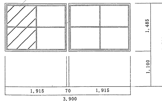
88号建物2階会議室 建具図 S=1/50
