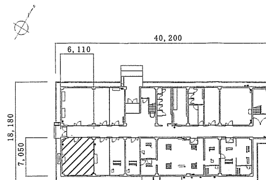
56号建物1階 平面図 S=1/500
