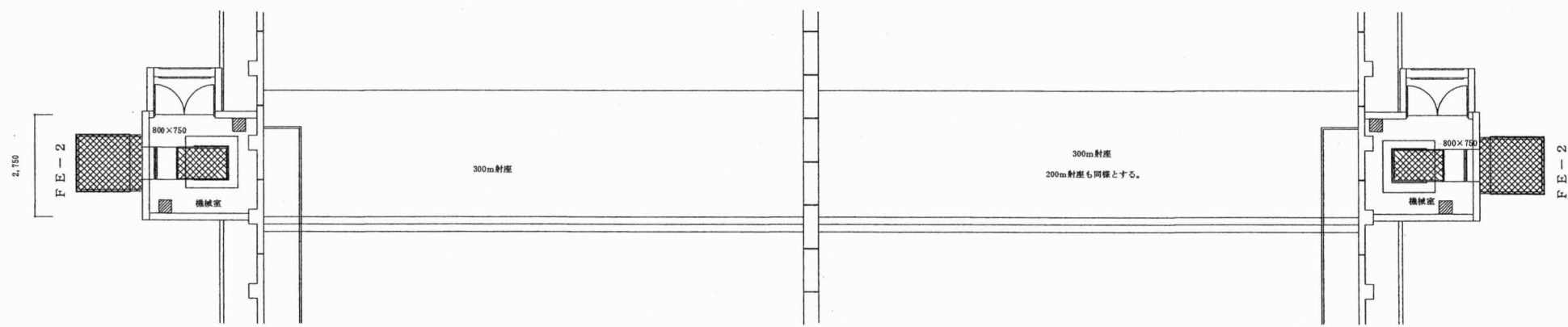
平面図 (300m射座) S=1/150
