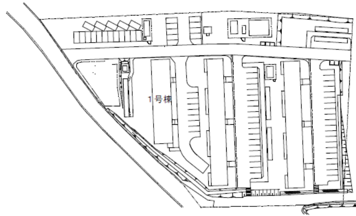
西岡宿舎配置図 S=1/700
