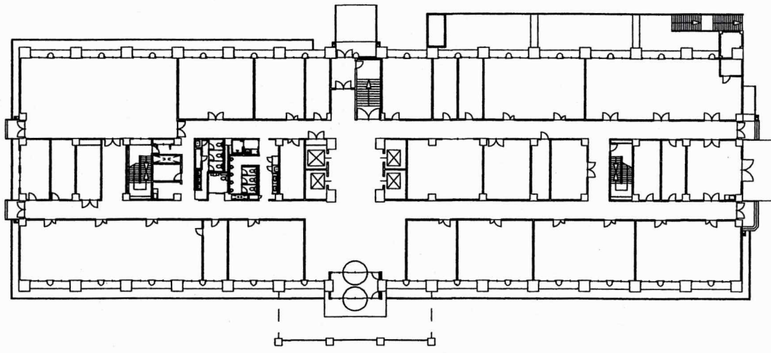
1号庁舎平面図 S = 1 : 1.5
