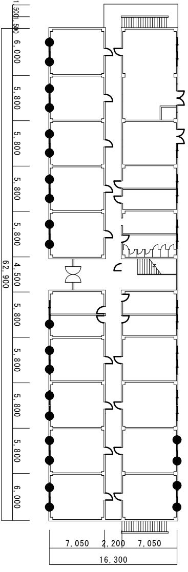
1511号建物1階平面図
