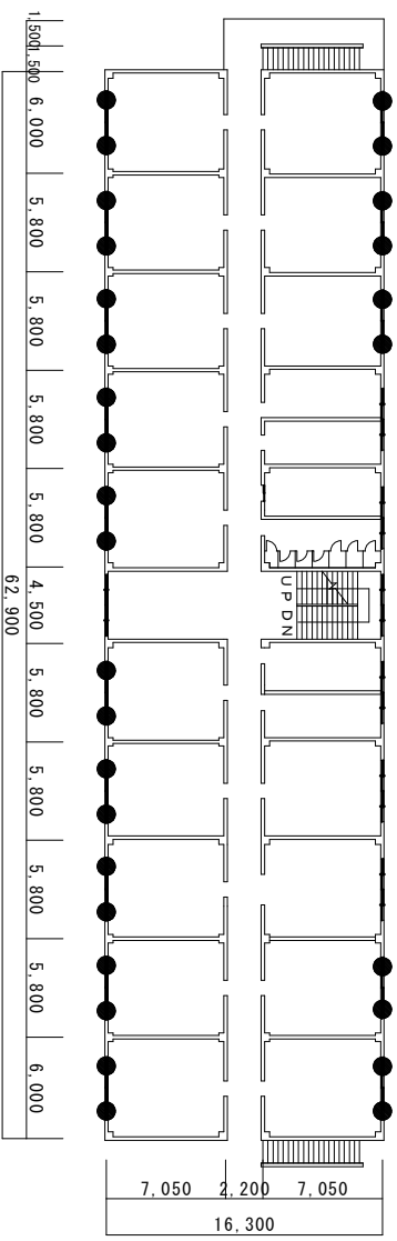
1511号建物2階平面図
