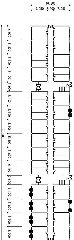
203号建物 1階平面図
