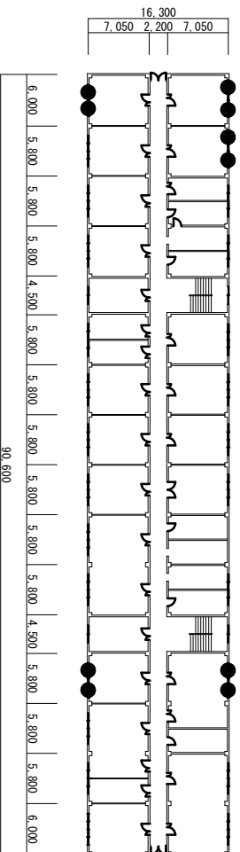
203号建物 2階平面図
