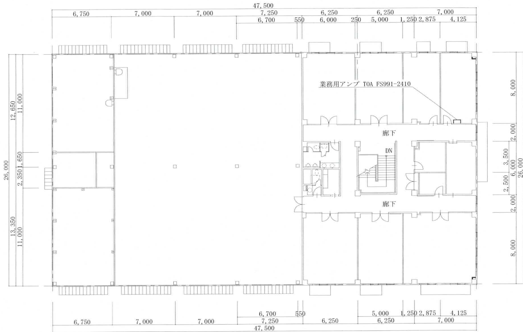
105号建物2F配置図 S=1/250
