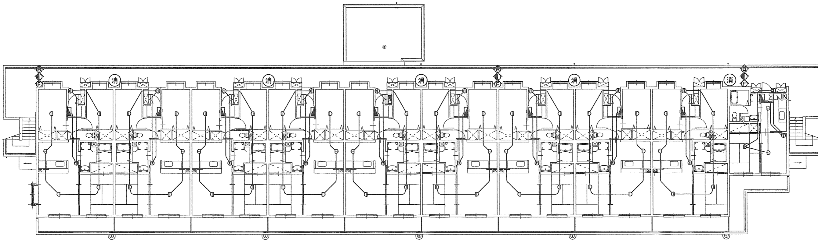
香我美宿舎A棟 2～5階消防設備図
