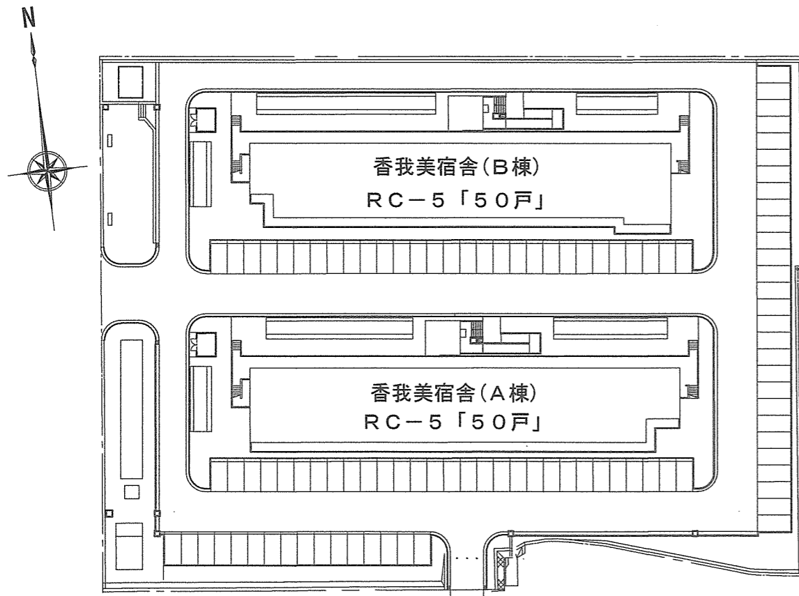
香我美宿舎配置図 S=1/800
