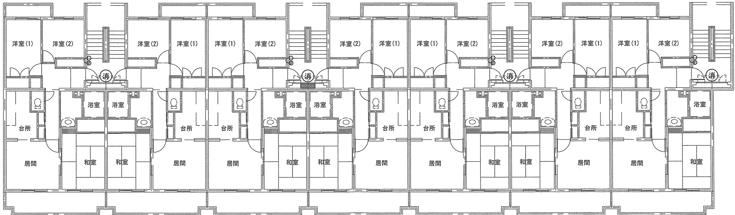
第2赤岡宿舎 1・3階消防設備図
