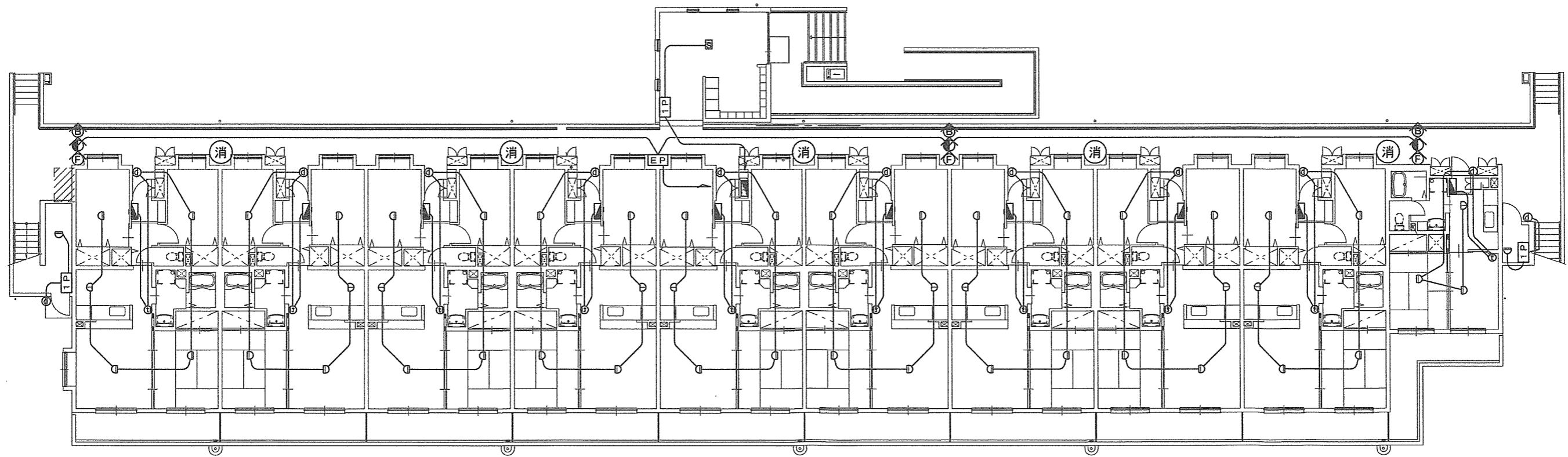
香我美宿舎A棟 1階消防設備図
