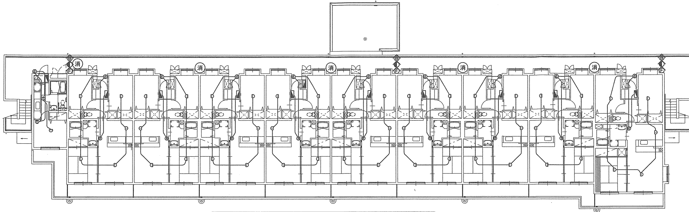
香我美宿舎B棟 2～5階消防設備図
