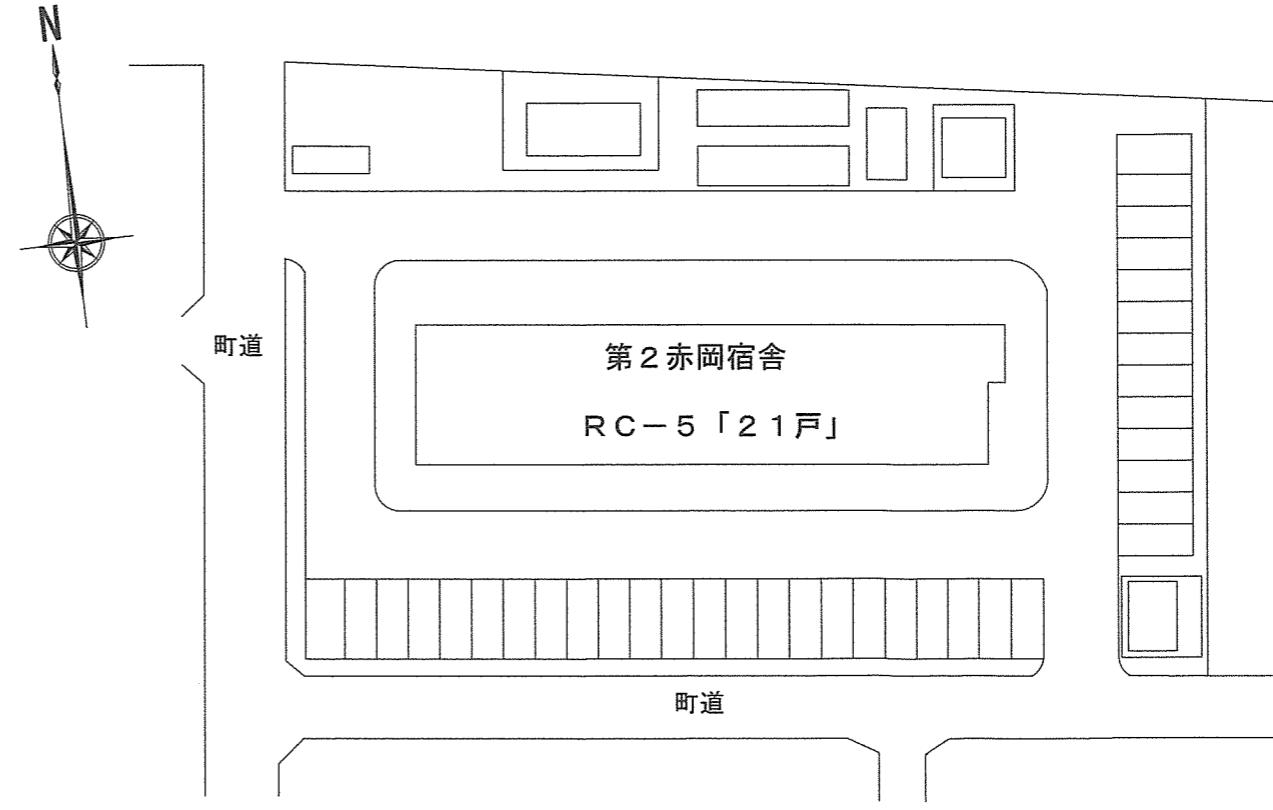
第2赤岡宿舎配置図 S=1/600
