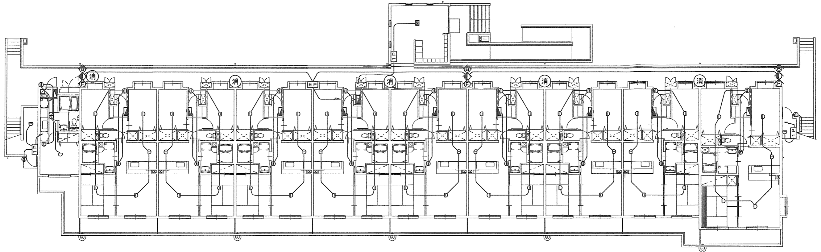
香我美宿舎B棟 1階消防設備図
