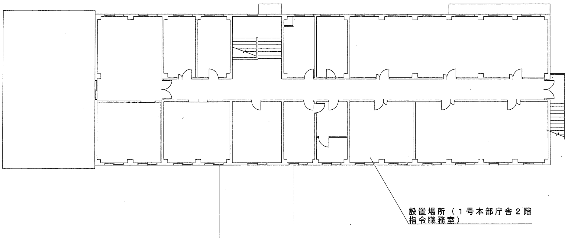
平面詳細図 (1/200)
