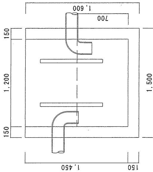
平面図
