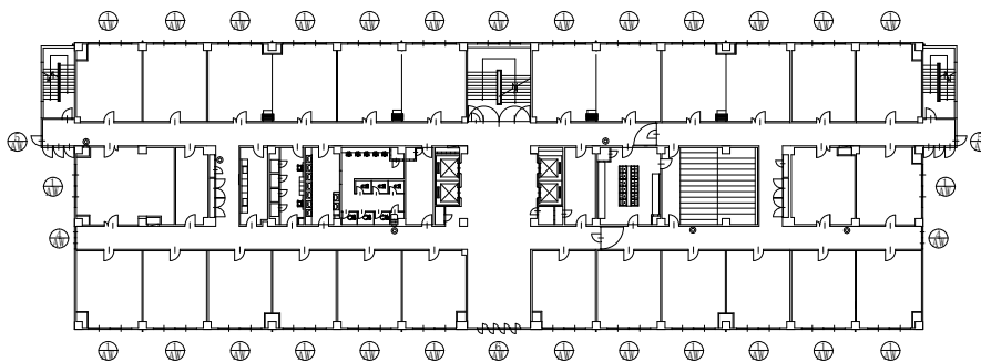
200号隊庁舎平面図
