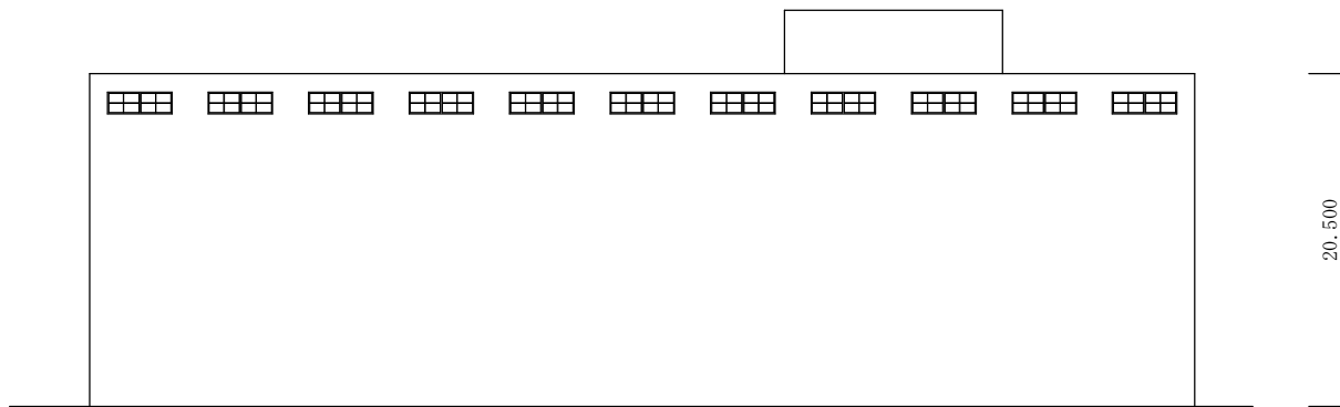
194号隊舎南側立面図
