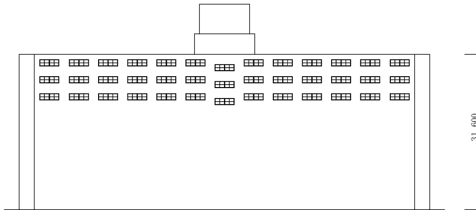
200号隊庁舎南側立面図
