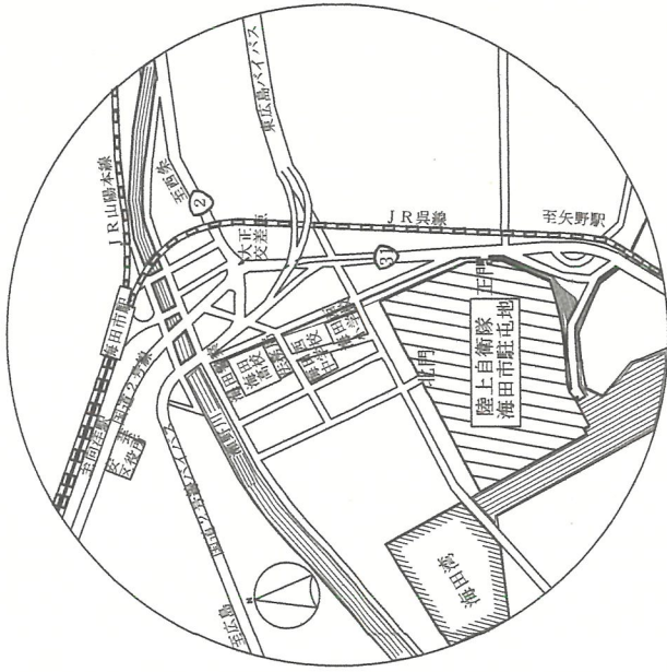
案内図 S = 1 / 4 5 0 0
