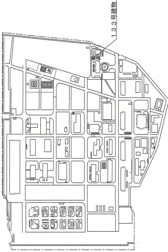
駐屯地配置図 S = 1 / 1 0 0 0
