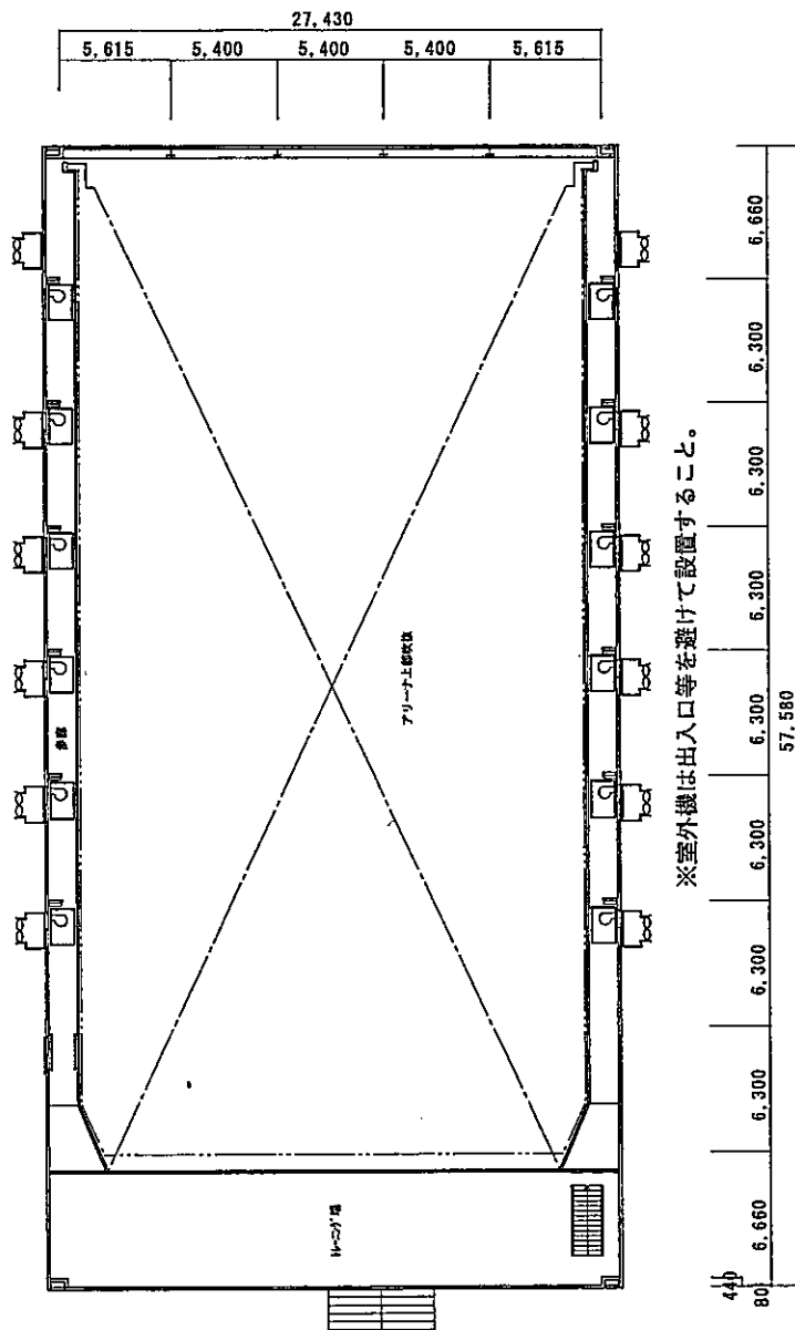
2階平面図 1/300
