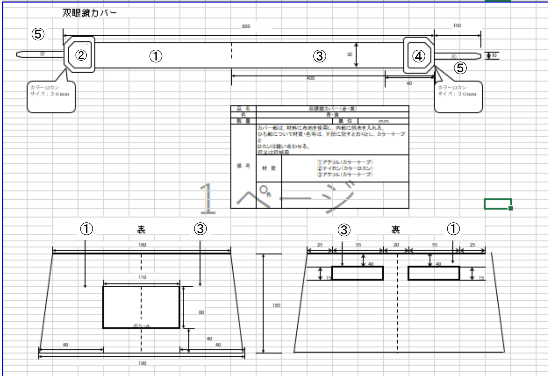
付図 2 - 形状及び寸法等
