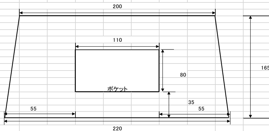
付図 3－形状及び寸法等
