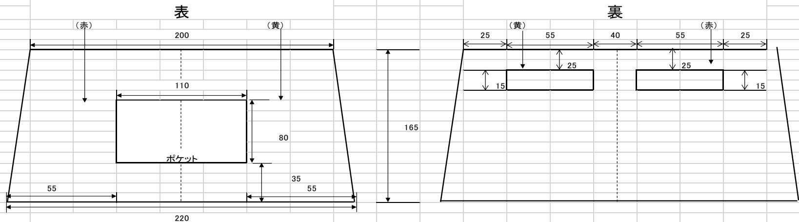
付図 2－形状及び寸法等
