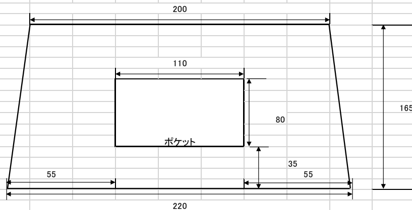
付図 6－形状及び寸法等
