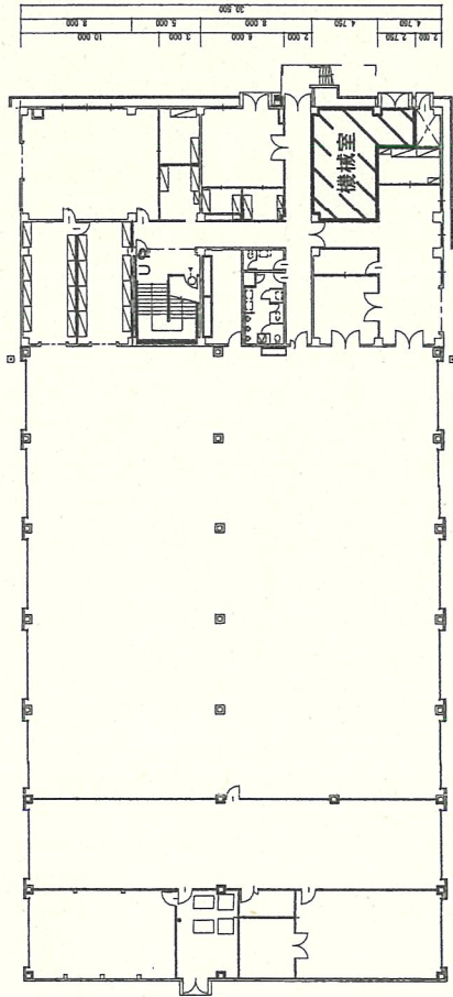
153号建物 1階平面図 (1/500)
