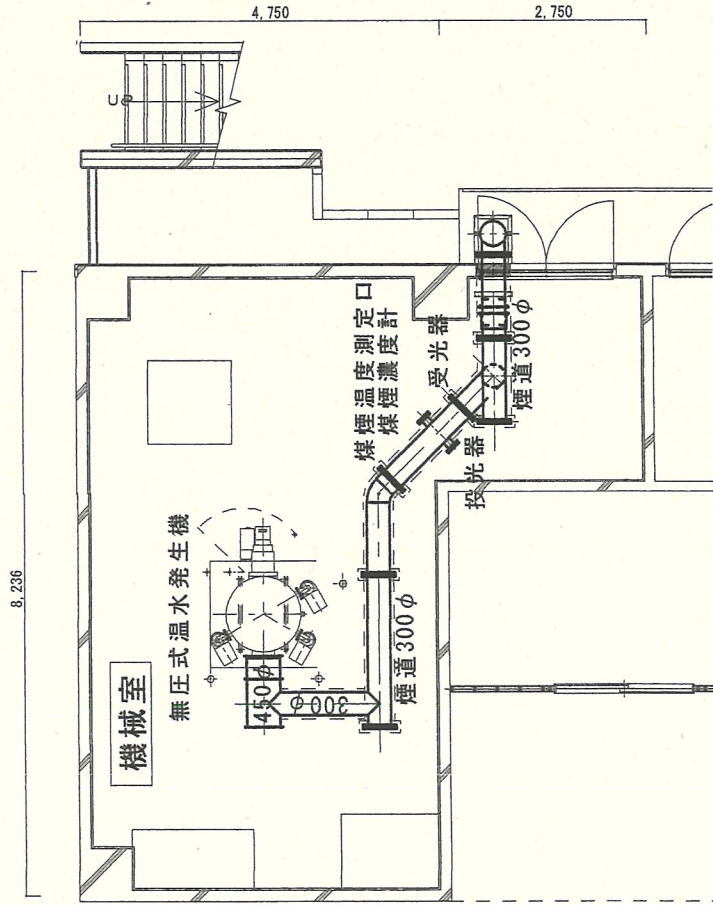
機械室平面詳細図 (1/100)
