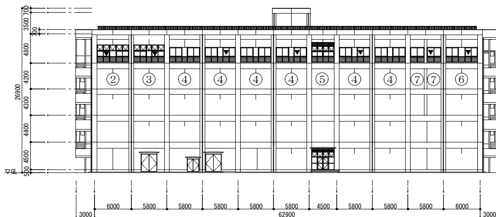
103号隊庁舎北側立面図
