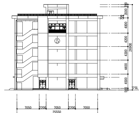
103号隊庁舎西側立面図
