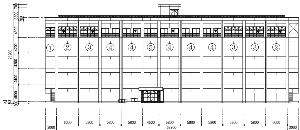
103号隊庁舎南側立面図
