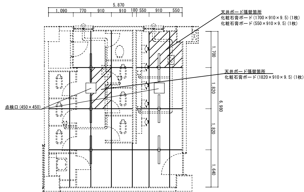
天井参考図 S=1/X
