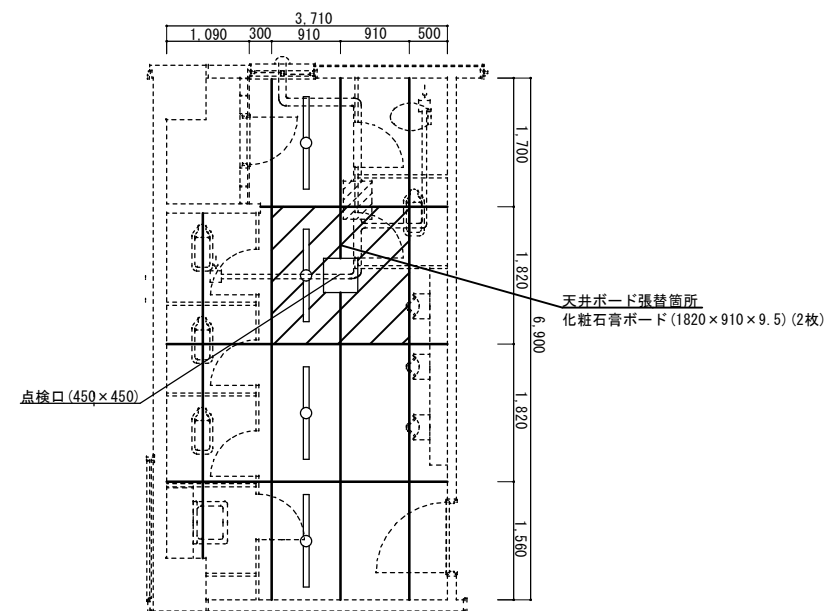
天井参考図 S=1/X
