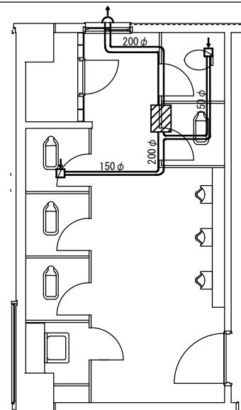
換気設備取替図 S=1/X
