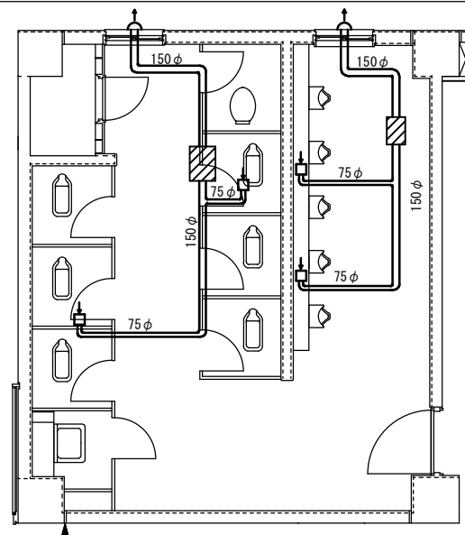
換気設備取替図 S=1/X
