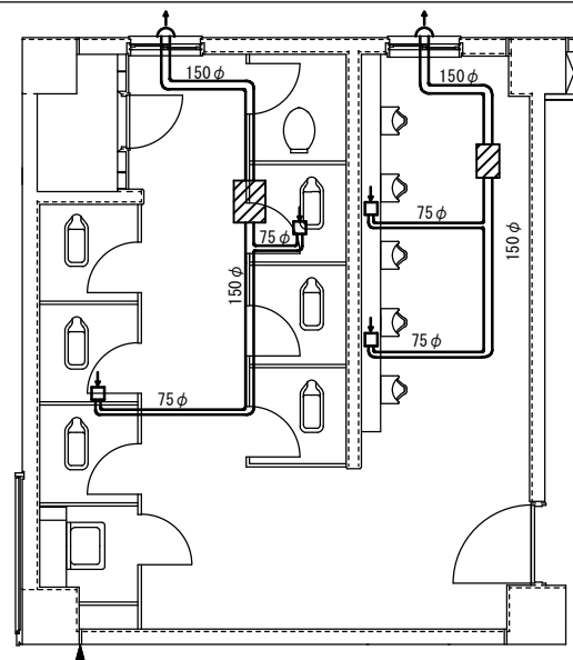
換気設備取替図 S=1/X
