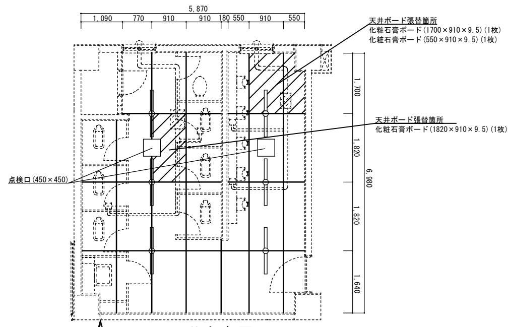
天井参考図 S=1/X
