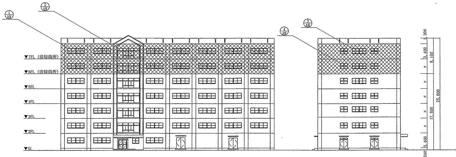
北側立面図
