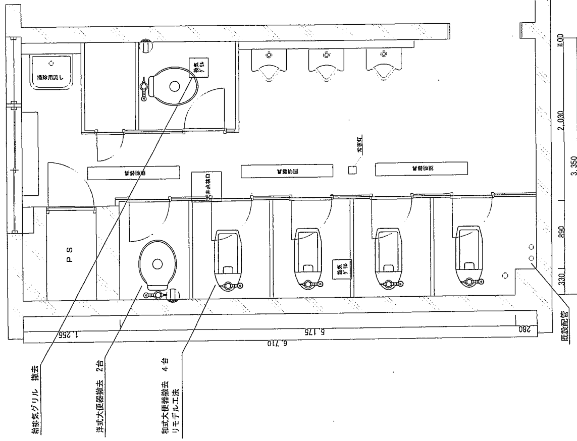
150号建物2階便所平面 既存図
