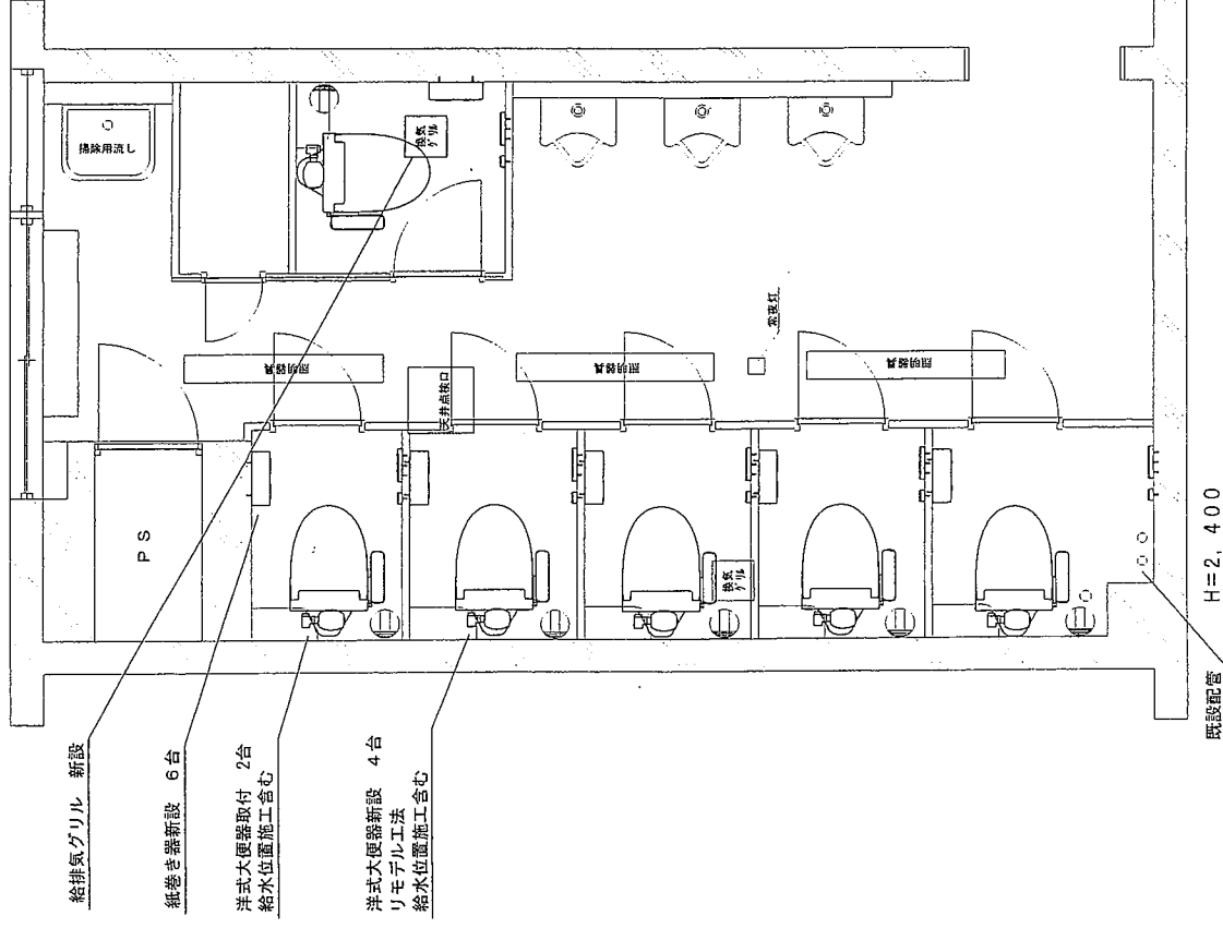
150号建物2階便所平面 改修図
