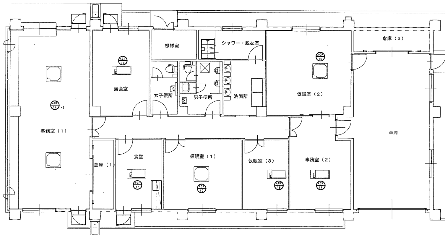
3号建物 1F空調設備配置図 1/100
