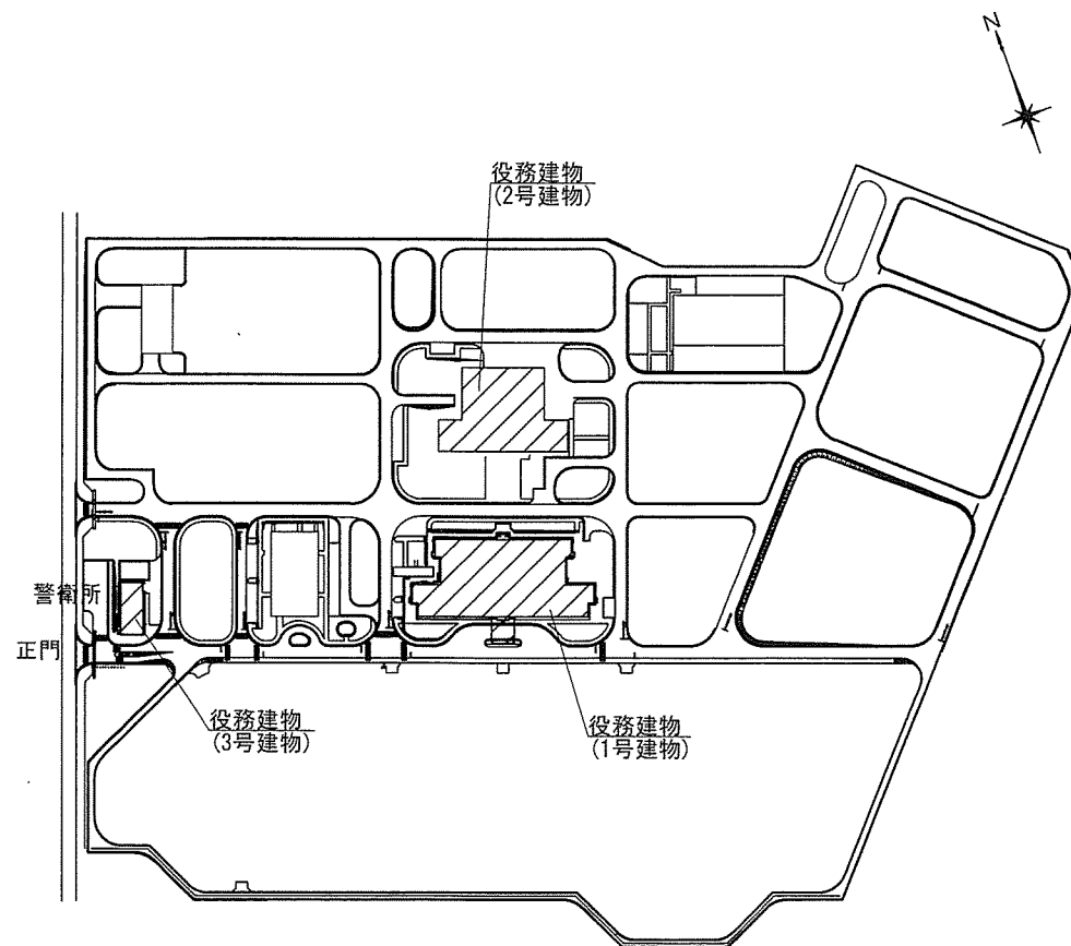
空調設備設置建物配置図
