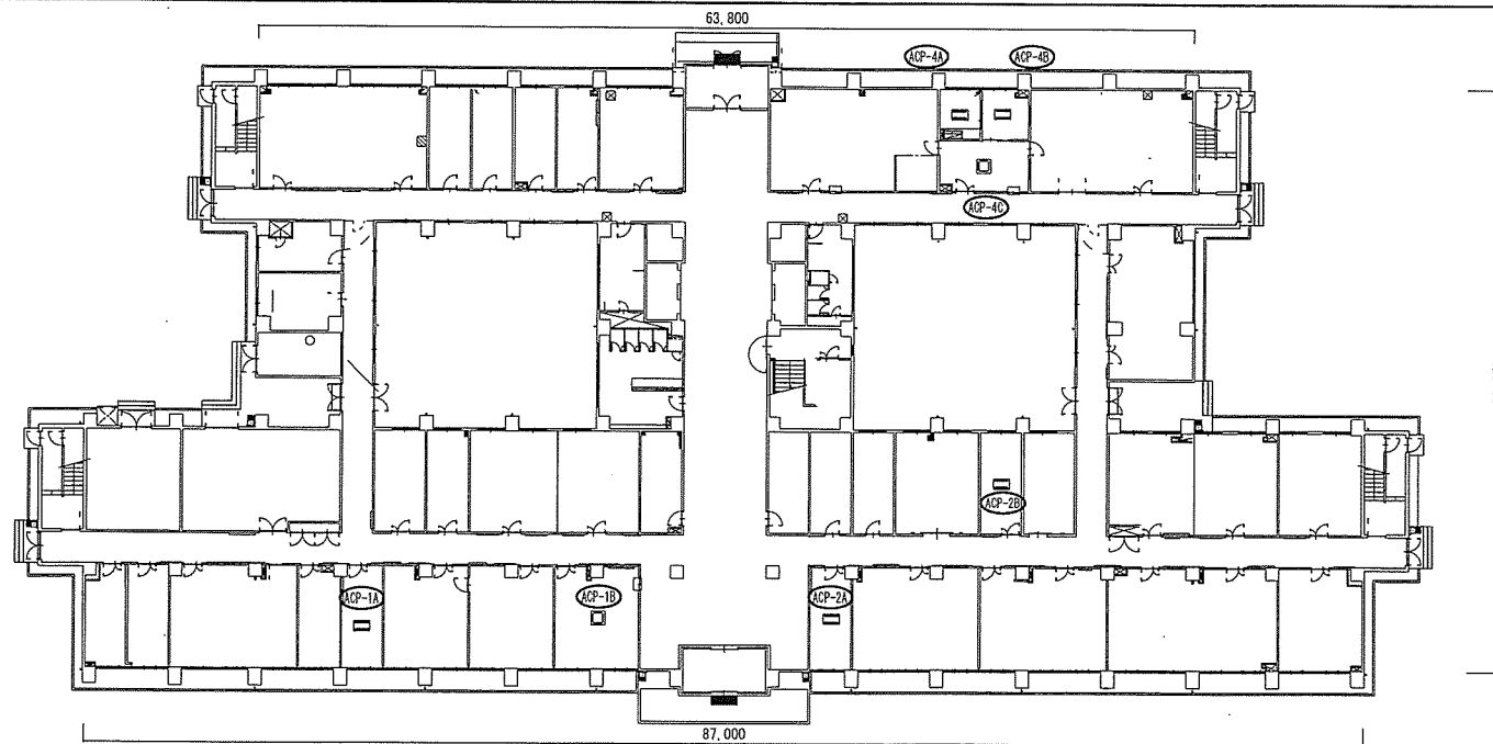
1号建物 1F空調設備配置図 1/400
