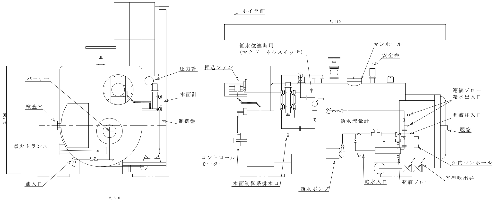
ボイラー立面図 1 : 3 0
