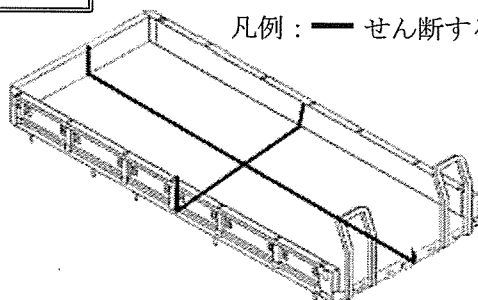
図4ー大型トラック外装部品及びフレームの解体・破碎図
