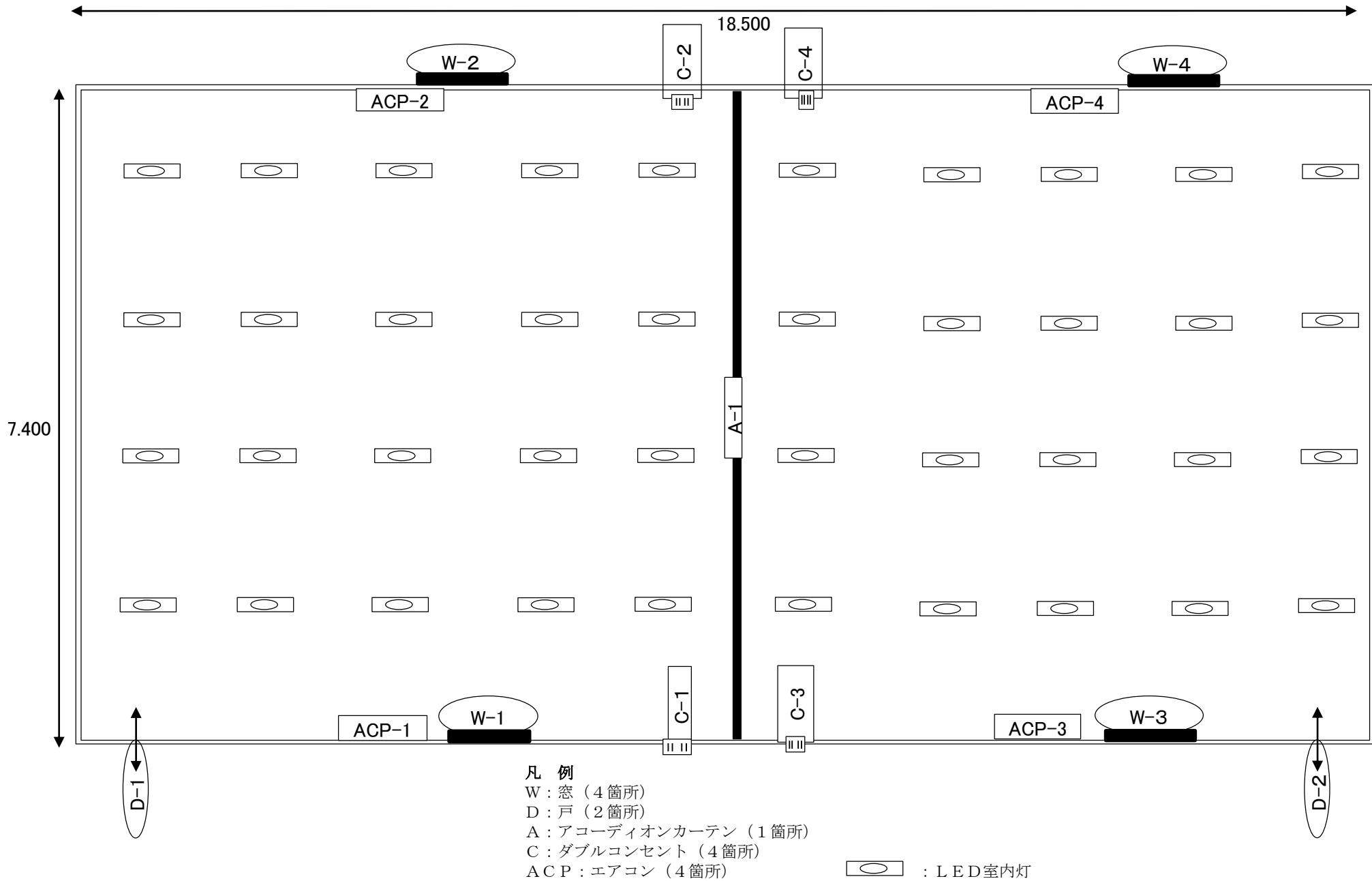
プレハブ平面拡大図
