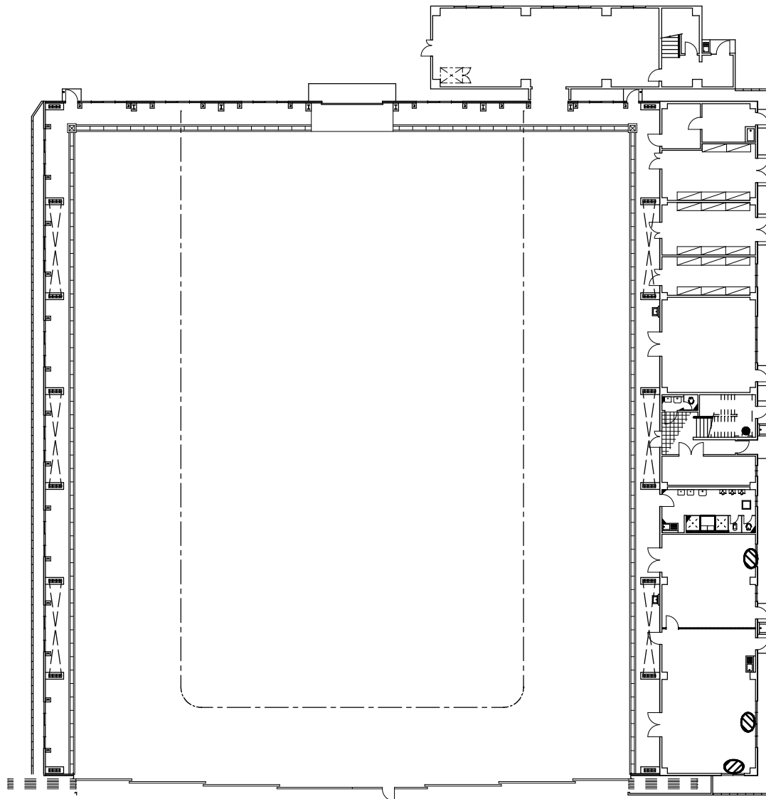
60号建物1F平面図 窓枠 h=1.6m
