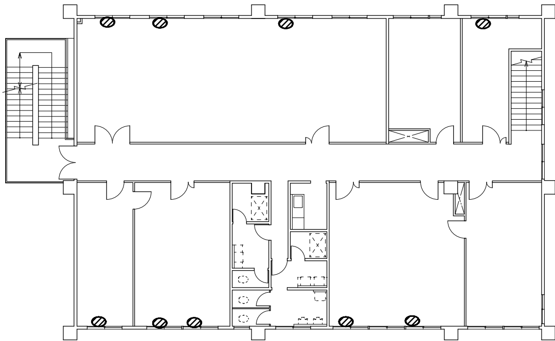
67号建物2F平面図 窓枠 h=1.6m
