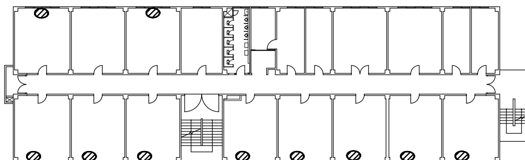
4号建物 3 F 平面図 窓枠 h=1.8m
