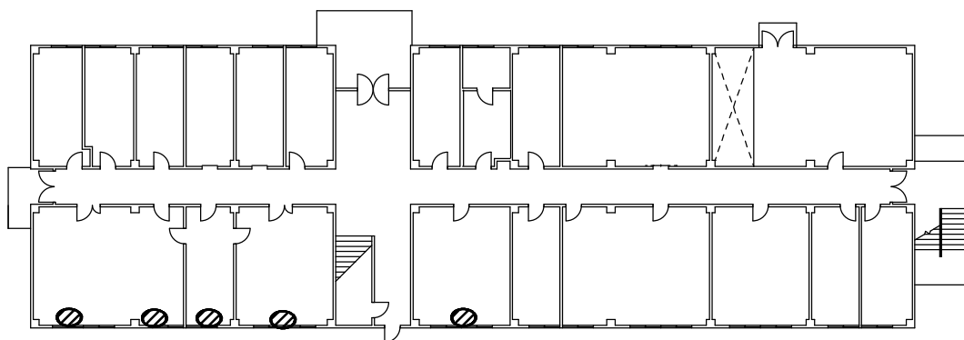
4号建物 1 F 平面図 窓枠 h=1.8m
