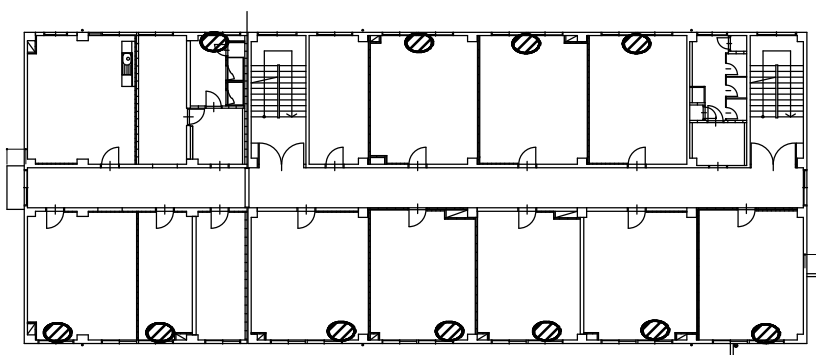
3号建物2F平面図 窓枠 h=1.8m
