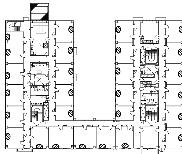
162号建物2F平面図 窓枠 h=1.3m
