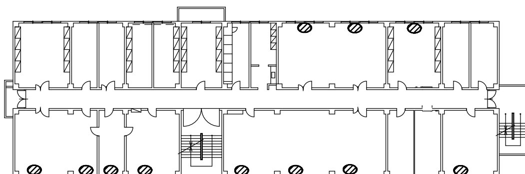
4号建物 2 F 平面図 窓枠 h=1.8m
