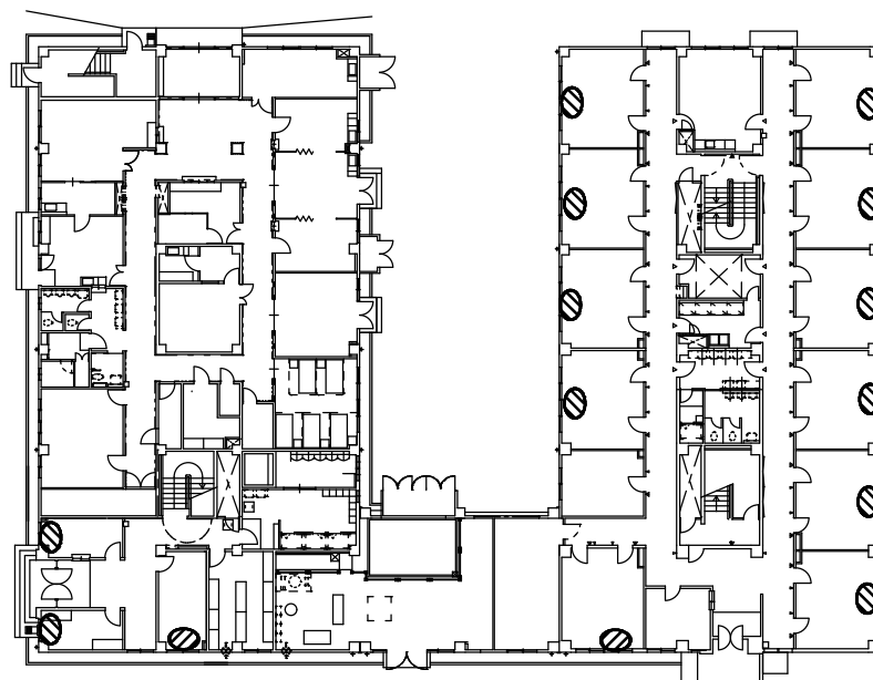
162号建物1F平面図 窓枠 h=1.3m
