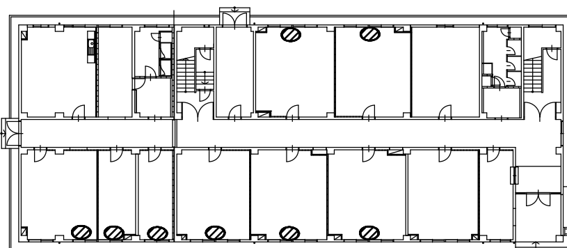
3号建物1F平面図 窓枠 h=1.8m
