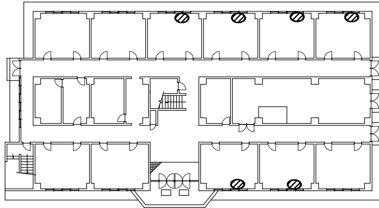
6号建物 1 F 平面図 窓枠 h=1.3m
