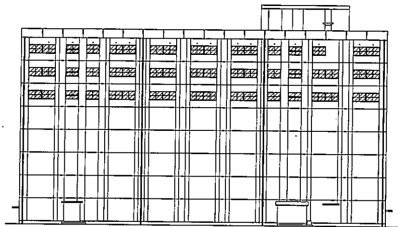
271号建物北侧立面图 S=1:400
