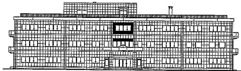
290号建物南側立面図 S=1:400
