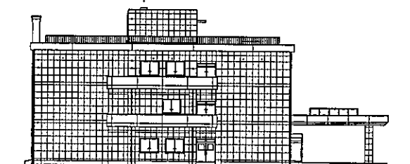
290号建物西側立面図 S=1:400
