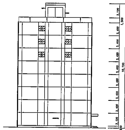
271号建物东侧立面图 S=1:400
