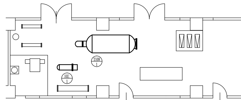
177号建物機械室平面図 S=1/100
