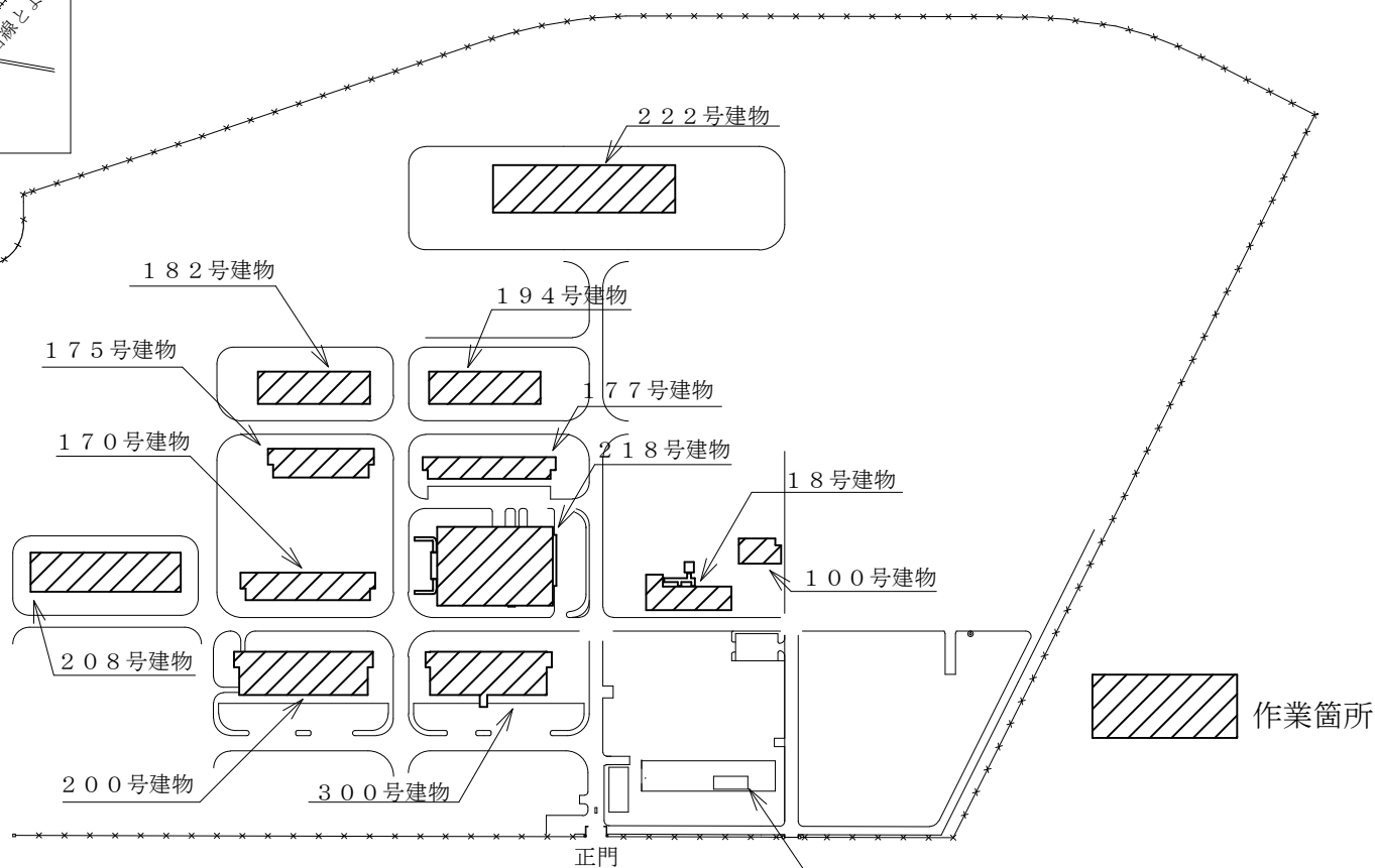
陸上自衛隊豊川駐屯地配置図 S : 1 / 4500
