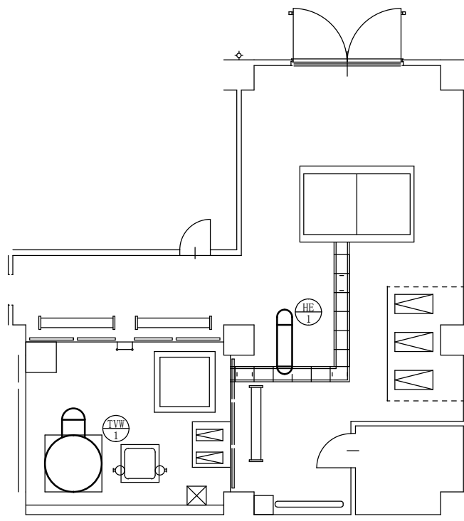
194号建物機械室平面図 S=1/100
