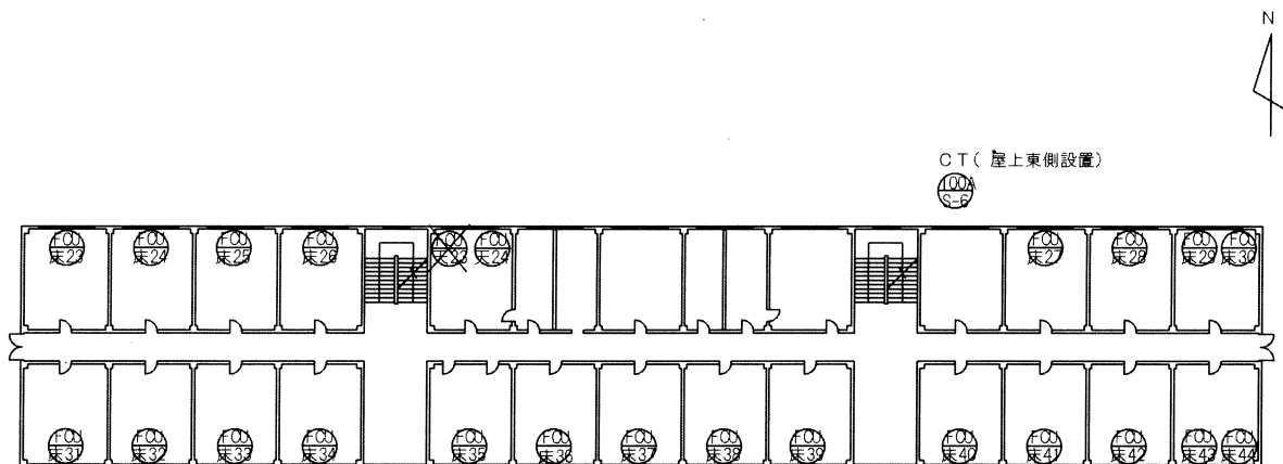
3 階平面図
