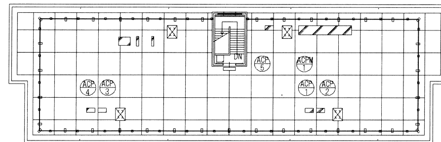
R階平面図
