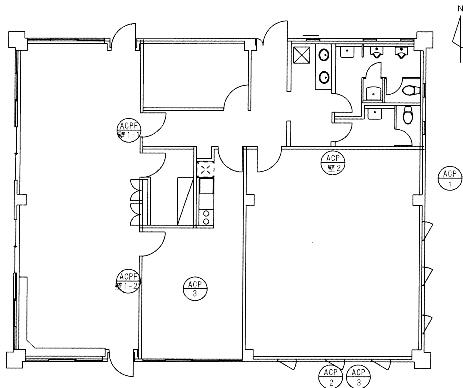
1 階平面図
