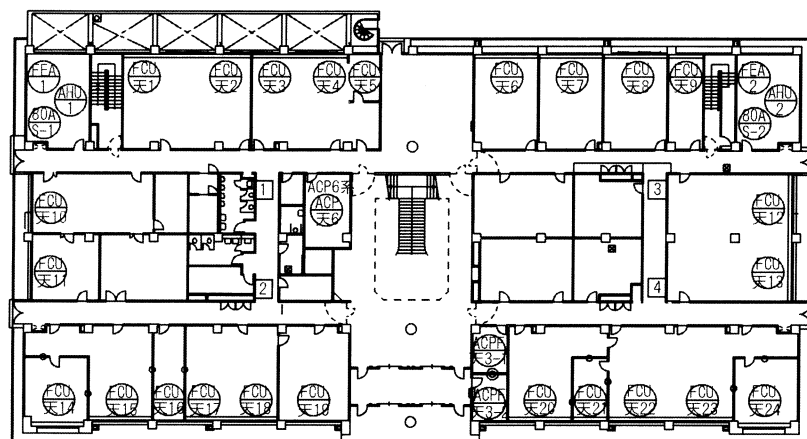
1階平面図
