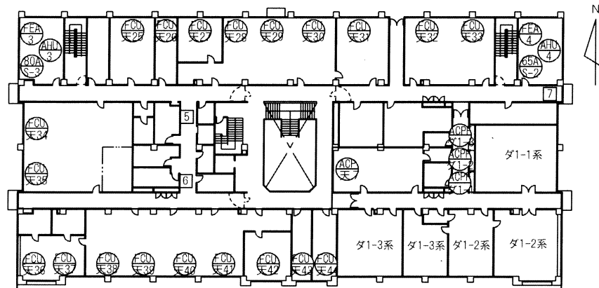
2階平面図
