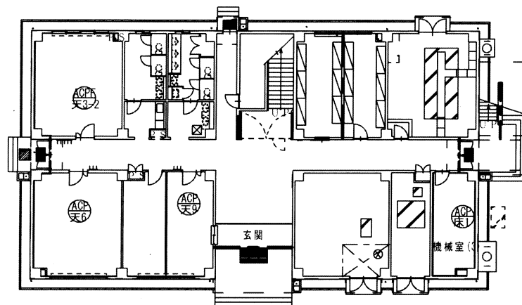
1階平面図
