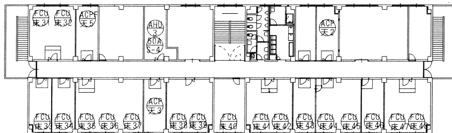
3 階平面図
