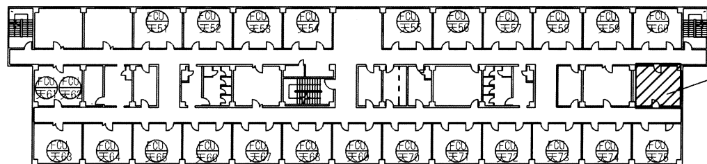
3階平面図
