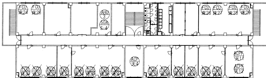
3階平面図
