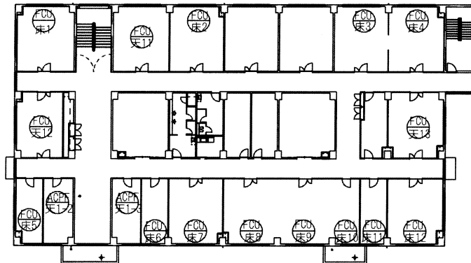
2階平面図
