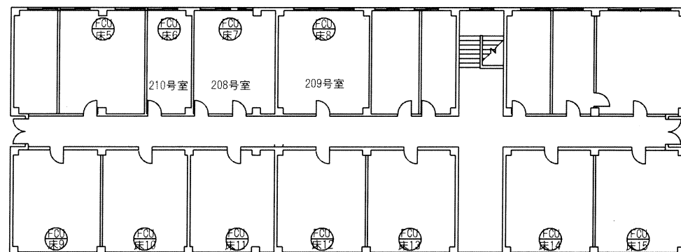
2 階平面図
