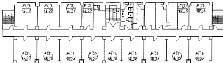
3階平面図
