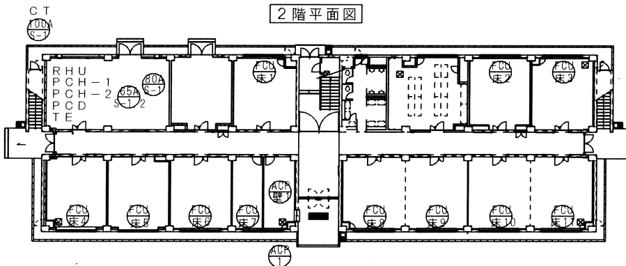
1 階平面図
