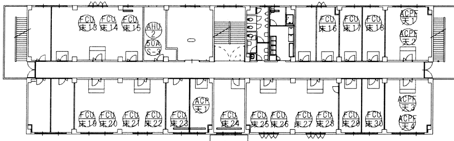
2 階平面図
