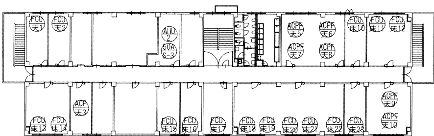
2階平面図
