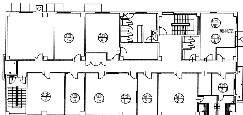
2階平面図
