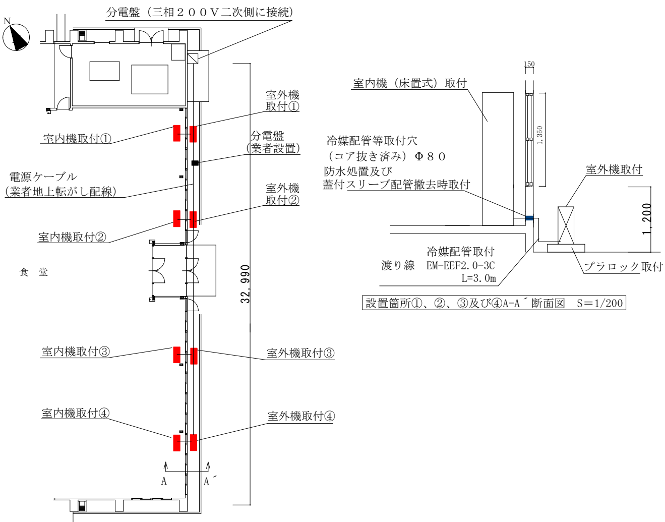
設置箇所イ 平面図 S=1/600
