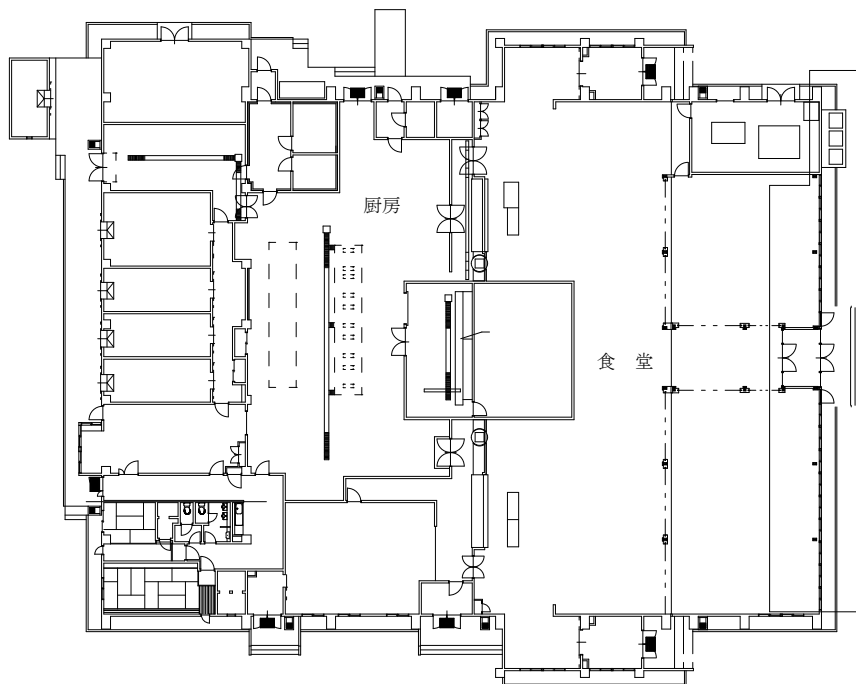
133号建物平面図 S=1/600
