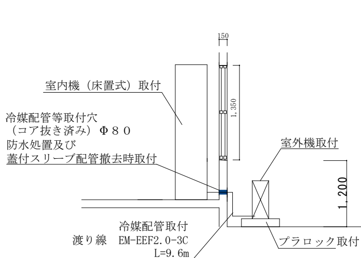
設置箇所アA-A断面図 S=1/200
