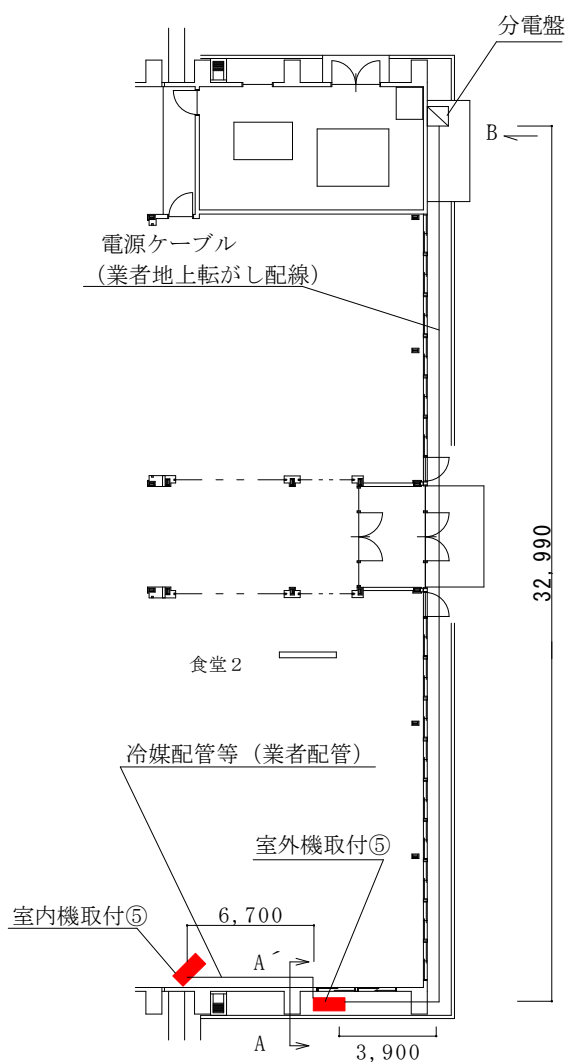
設置箇所ア平面図 S=1/600
