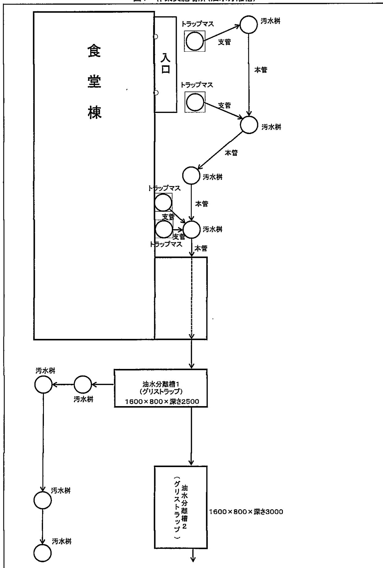
図1—作業実施場所(油水分離槽)
