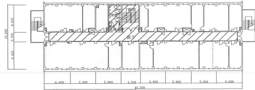
30号建物3階平面図 S=1:X
