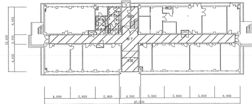
30号建物1階平面図 S=1:X
