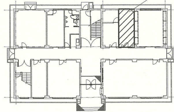
64号建物1階平面図 S=1/400
