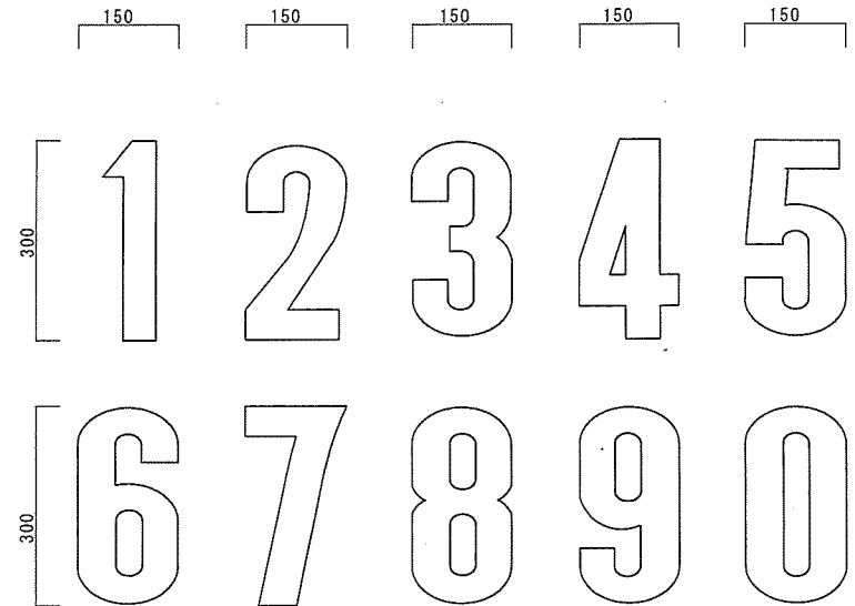
路面標示詳細図 S = 1 / 25
