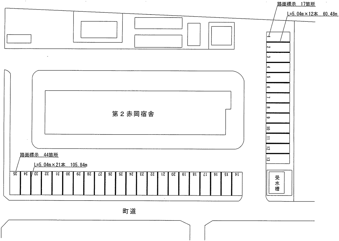
第2赤岡宿舎配置図 S=1/400
