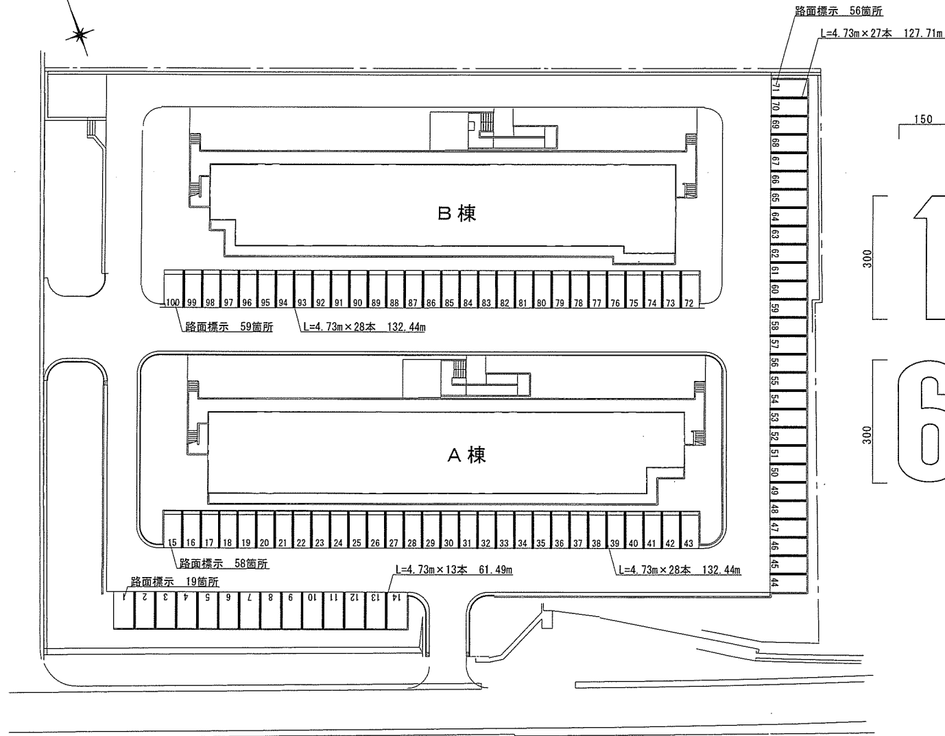
香我美宿舎配置図 S = 1 / 75
