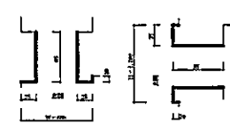
WD6平面・断面詳細図 6/23
