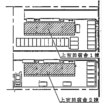
上吉田宿舎配置図 S=1/1,000
