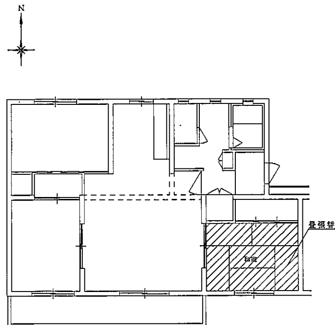
生野宿舍1棟 (D規格) 施工平面図 S=1/100
