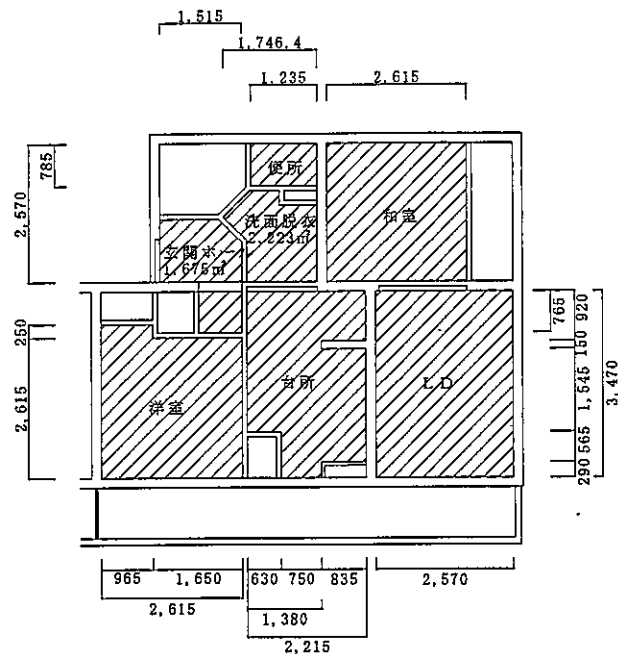
上吉田宿舎 1・2棟.c規格 天井伏せ図 S=1/100
