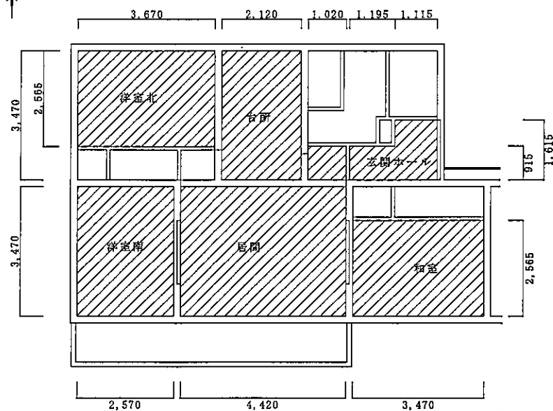
生野宿舎1棟d規格 天井伏せ図 S=1/100
