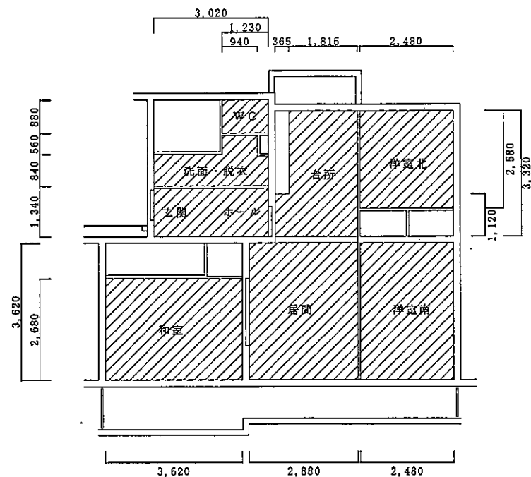
生野宿舎2棟c規格 天井伏せ図 S=1/100
