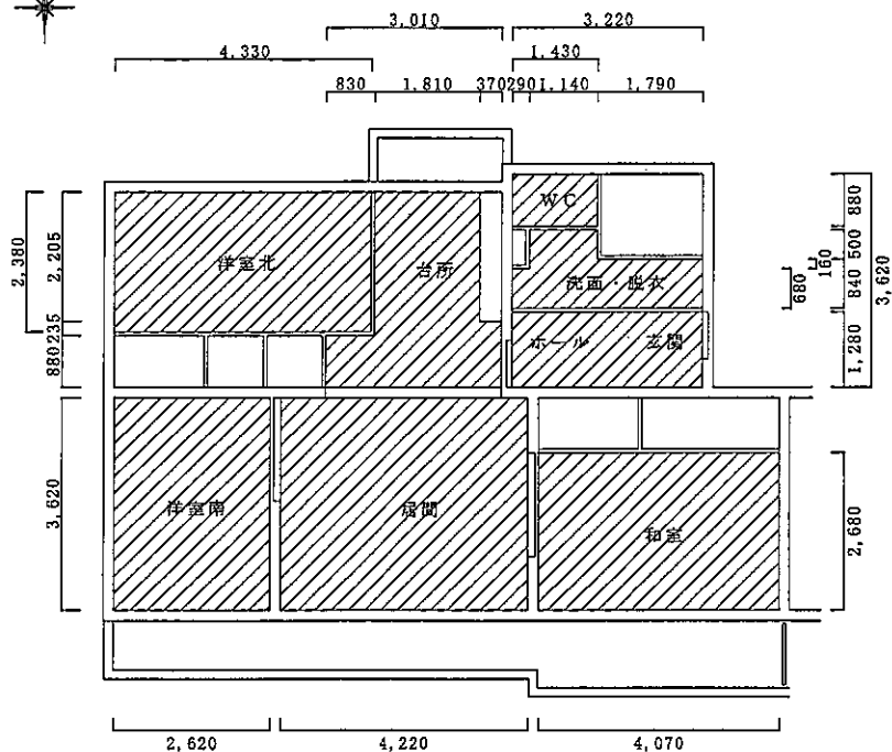
生野宿舎 2棟.d規格 天井伏せ図 S=1/100
