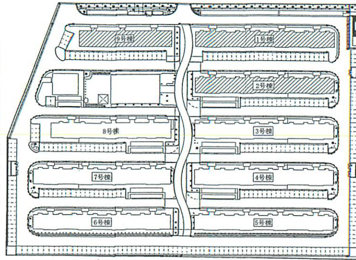
配置図
