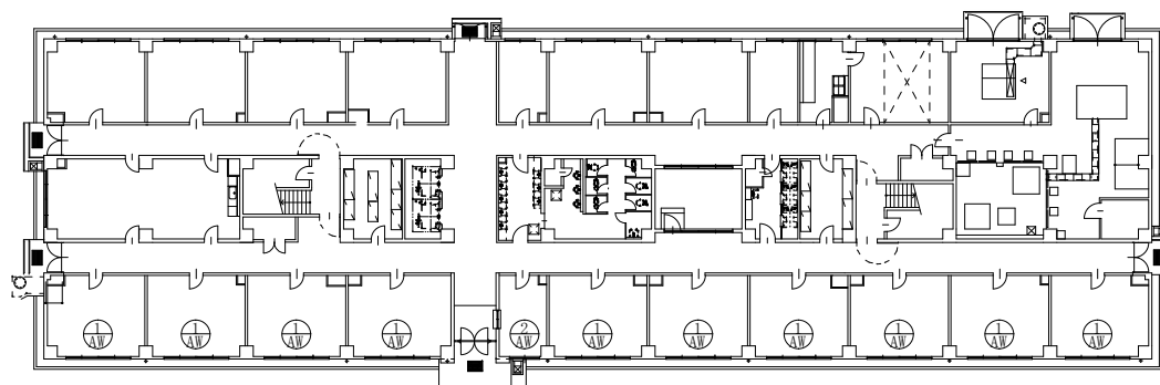
194号隊舎1階平面図
