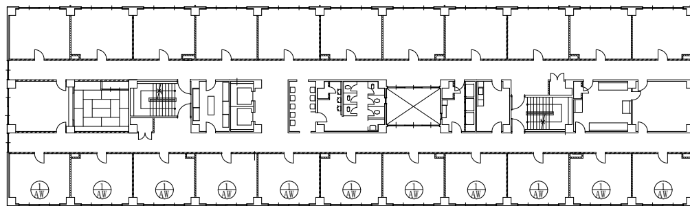
182号隊舎2～6階平面図
