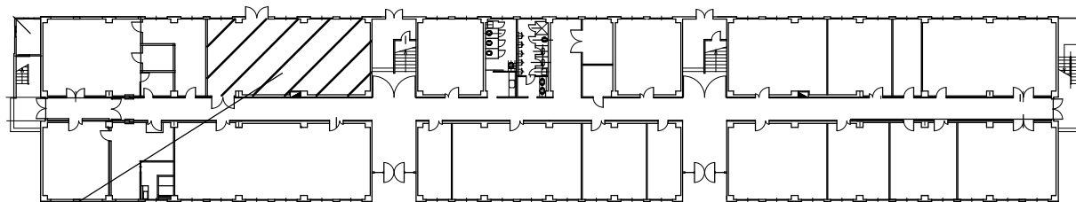
1号建物平面図 S=1/300
