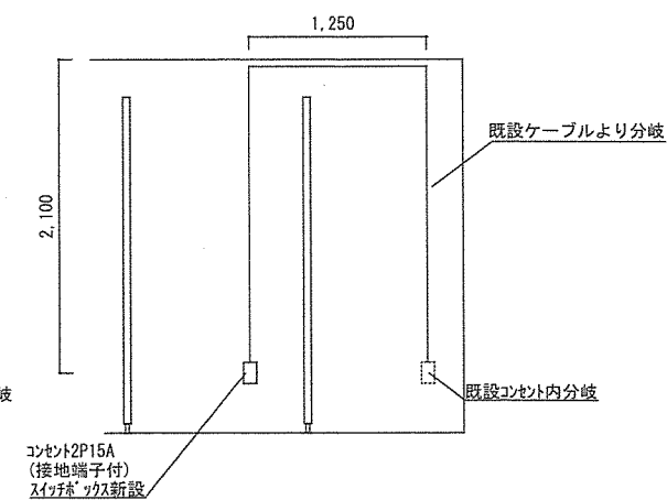
A-A' 展開図 1 : 30
