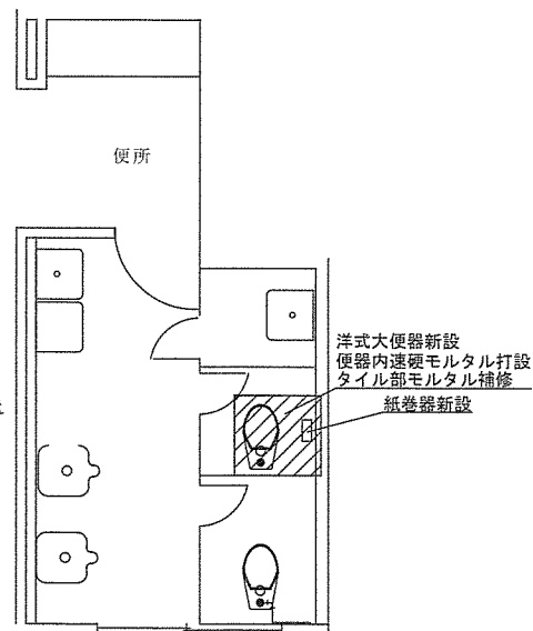
改修後詳細平面図 1 : 60
