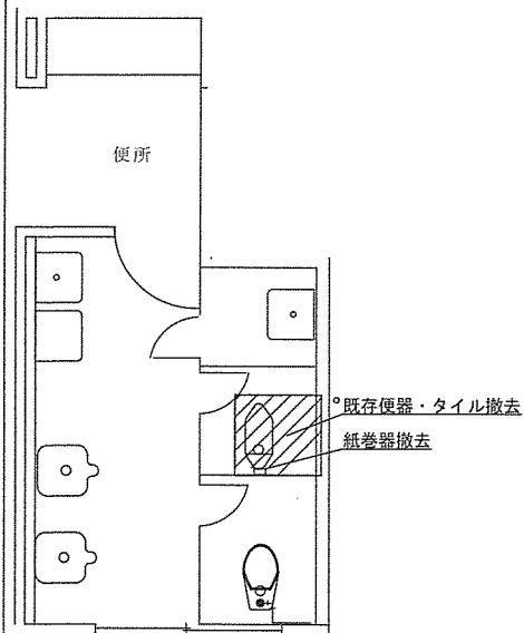
改修前詳細平面図 1 : 60
