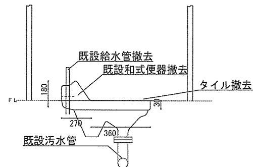
便器取替改修前標準詳細図 S = 1 : 15
