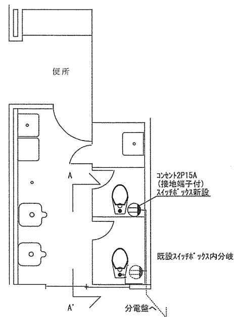
電気配線図 1 : 60
