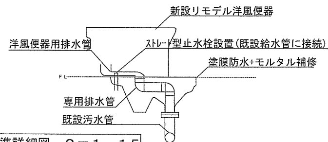
便器取替改修後標準詳細図 S = 1 : 15
