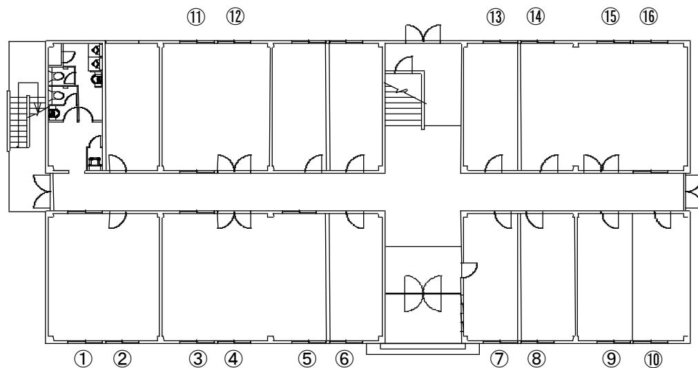
1号隊舎 1階平面図 S=1/250
