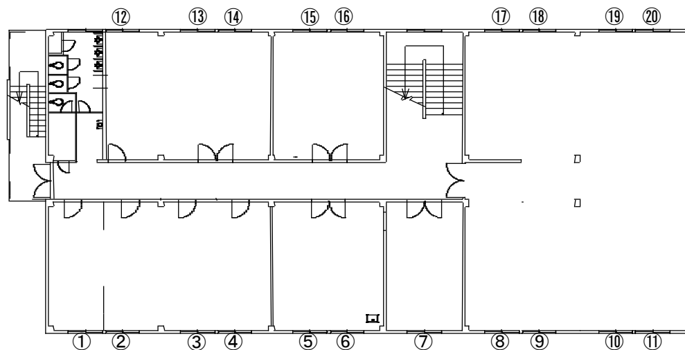
1号隊舎 2階平面図 S=1/250
