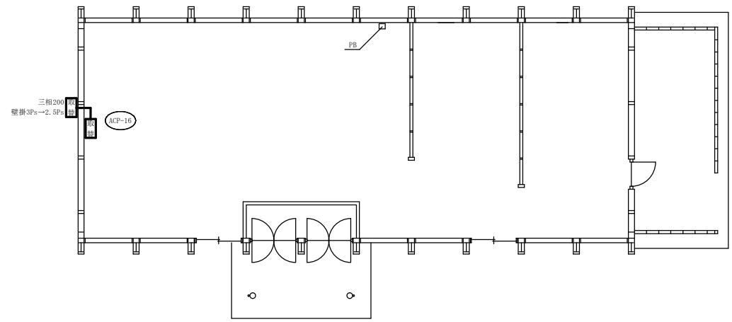
98号建物平面図 S/N
