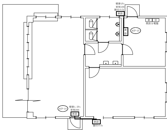
91号建物平面図 S/N
