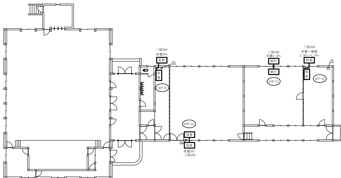
5号建物平面図 S/N
