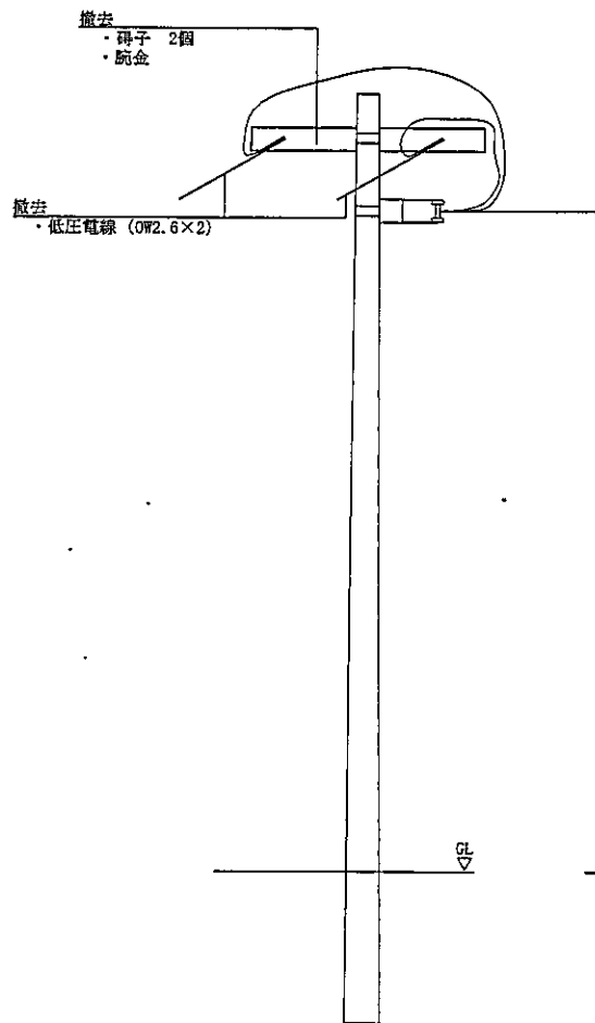
装柱撤去図
