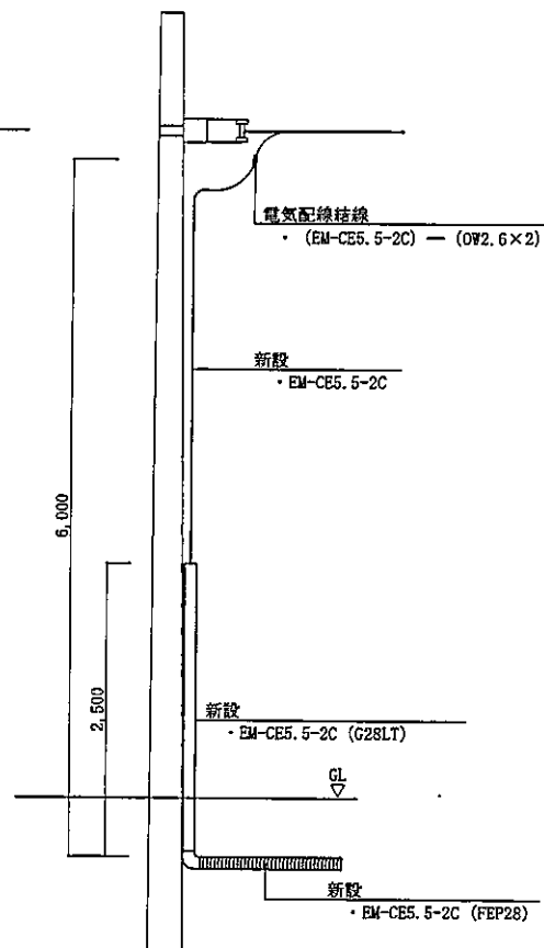
装柱新設図
