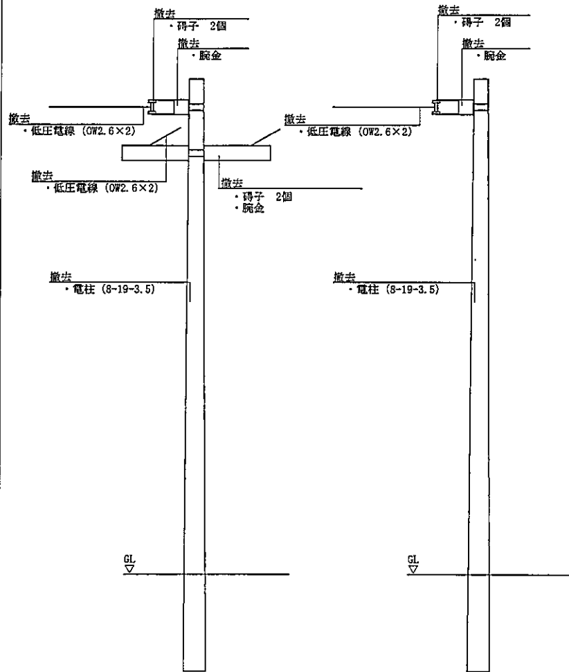
電柱標準図 (#2)
