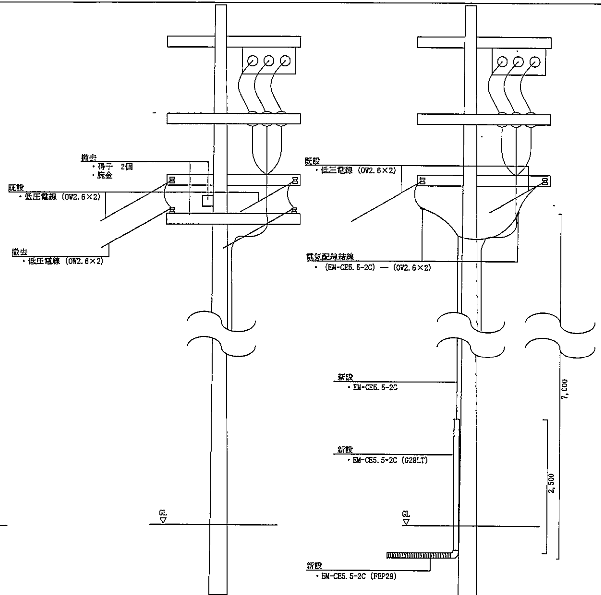
装柱撤去図
