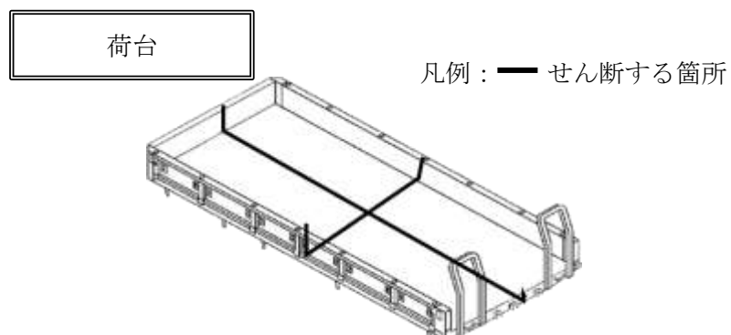
図2—中型トラック外装部品及びフレームの解体・破碎図
